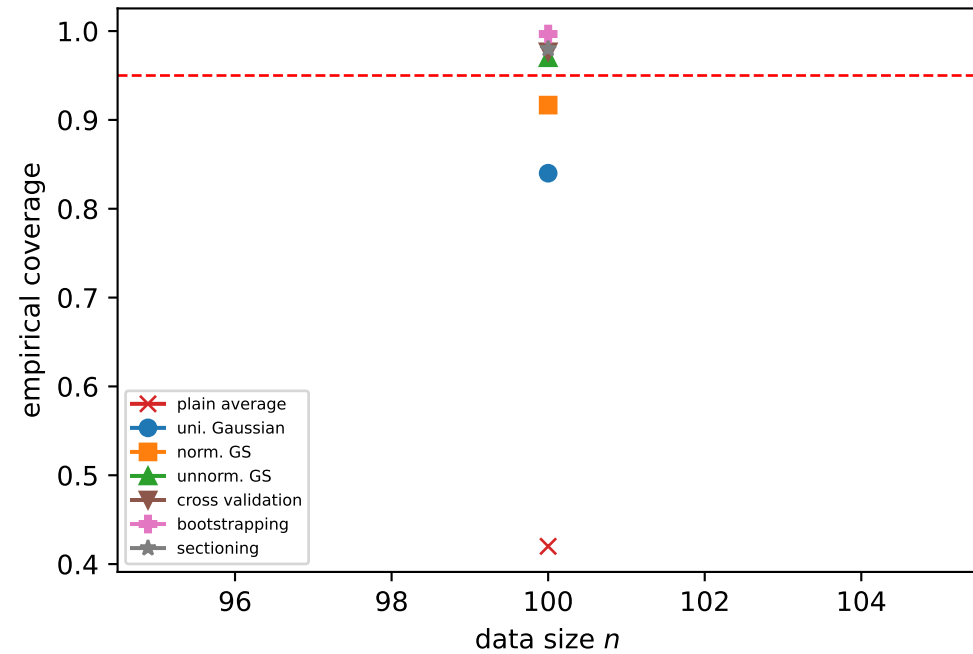
paper_dro_wasserstein (split=0.7)
