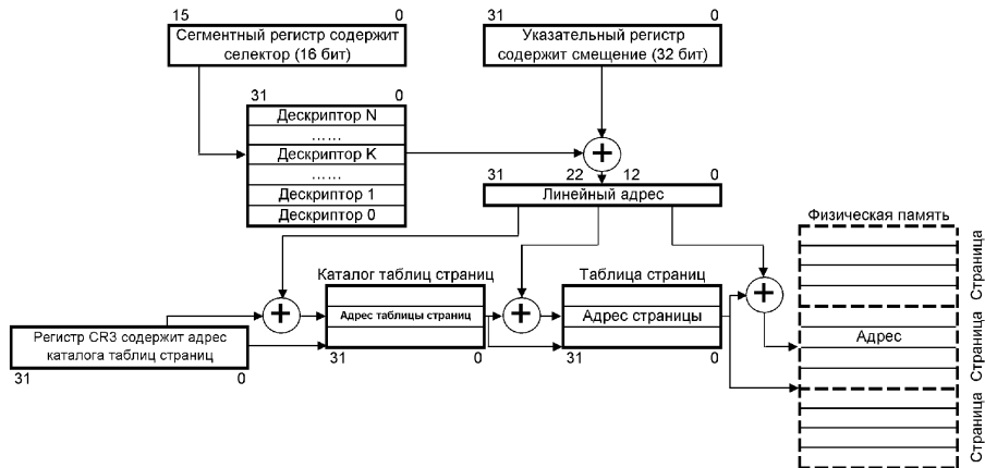
Адресное преобразование 80386
