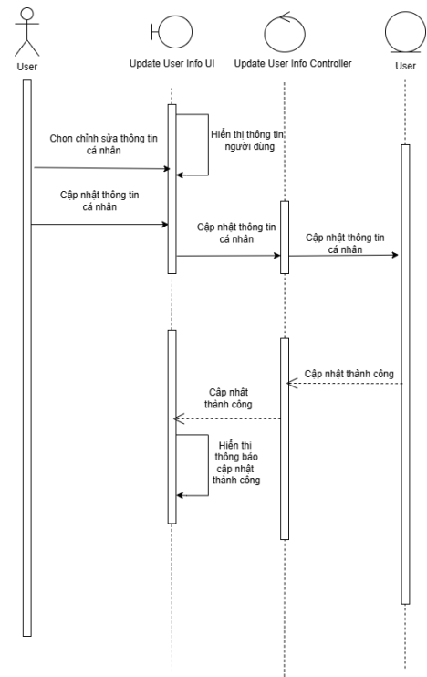
Hình 7: Biểu đồ tuần tự ca sử dụng chỉnh sửa thông tin cá nhân
