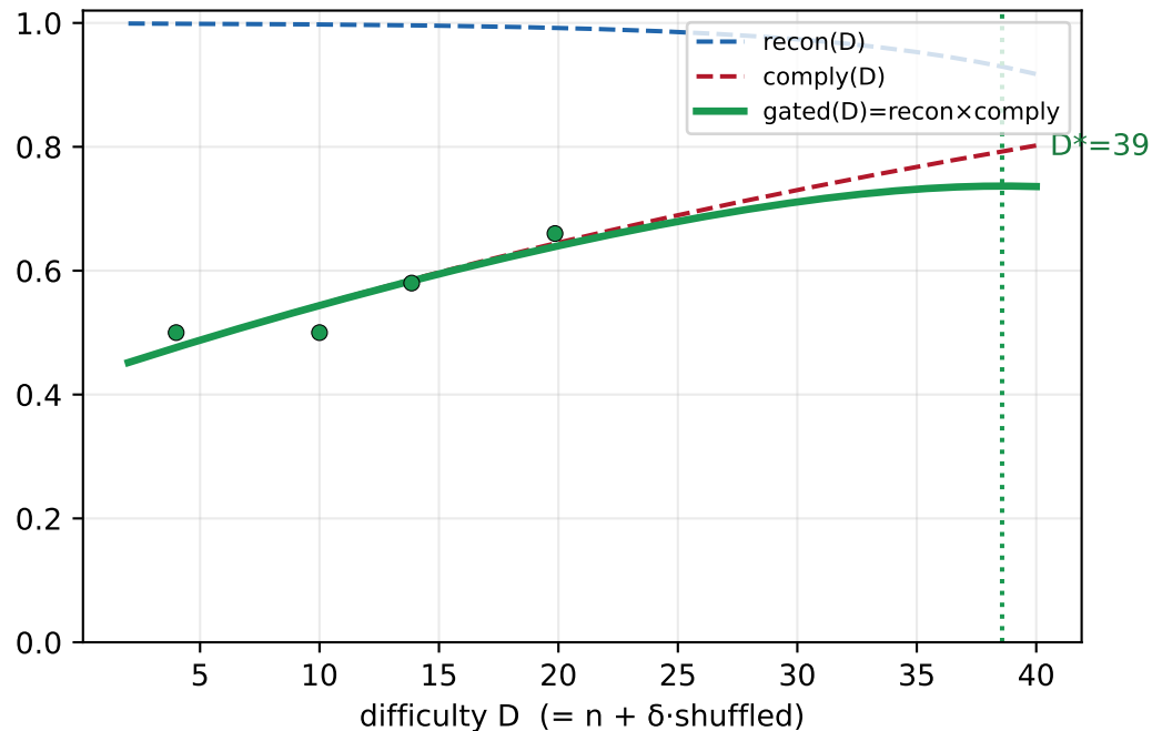
GPT-4o (stronger reconstructor)
