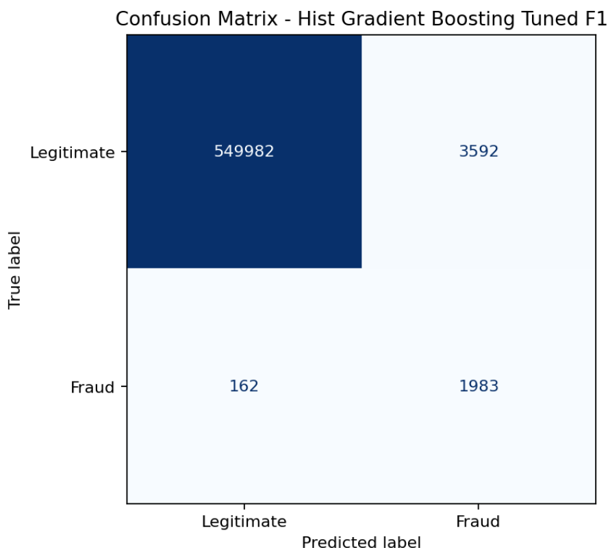
Hình 6: Confusion matrix của mô hình tốt nhất
