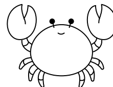
Cangrejo 27
