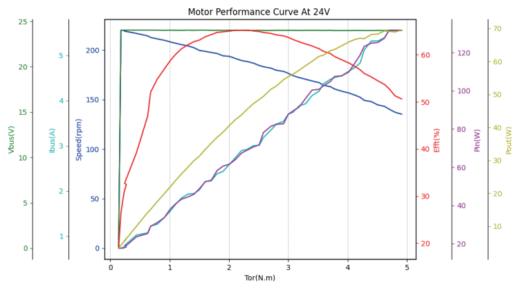
性能曲线 (Performance Curve)
