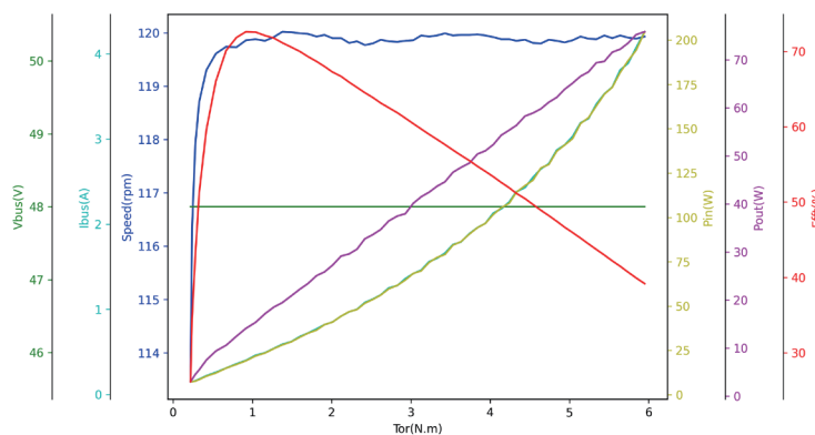
性能曲线 (Performance Curve)
