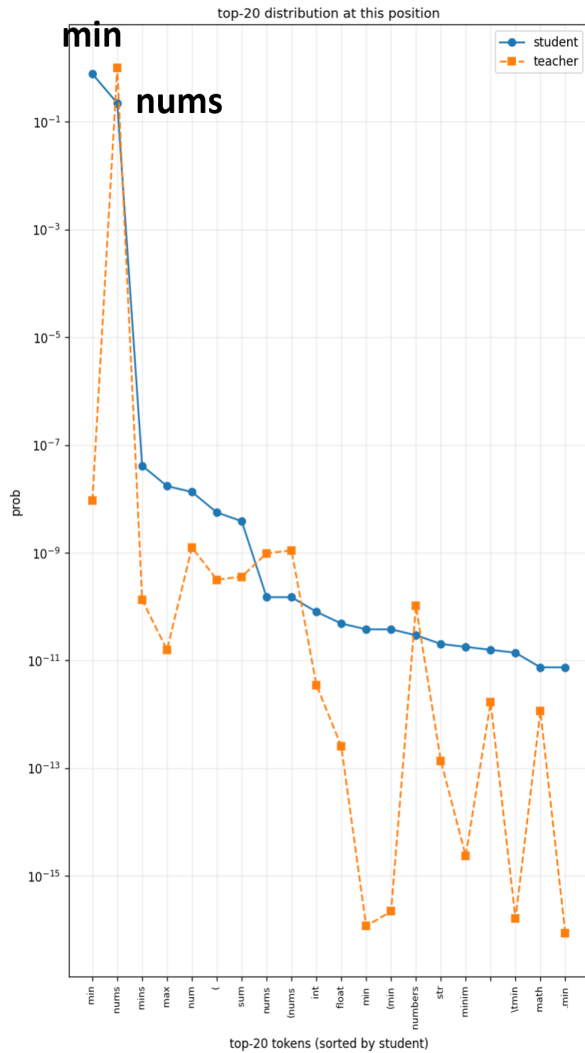
그림 5. 성공 rollout의 특정 토큰 위치에서의 student와 self-teacher 분포 비교 x축은 student의 확률 기준으로 정렬된 top-20 토큰 후보를, y축은 각 토큰의 확률을 나타낸다. 파란색은 student 분포를, 주황색은 self-teacher 분포를 나타낸다.
