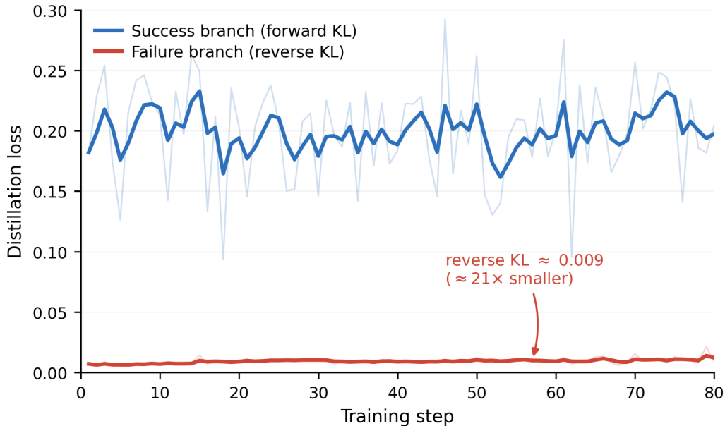
그림2. 학습 중 성공 분기와 실패 분기의 증류 손실 변화
