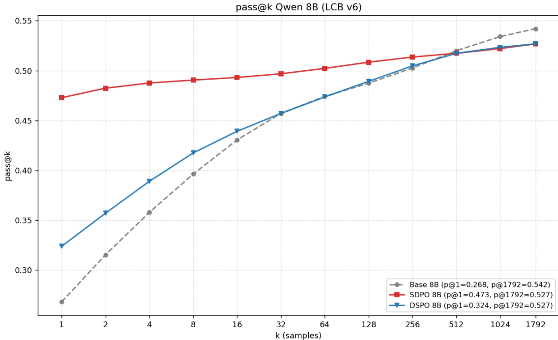
그림1. Qwen3-8B의 LiveCodeBench v6 pass@k 곡선
