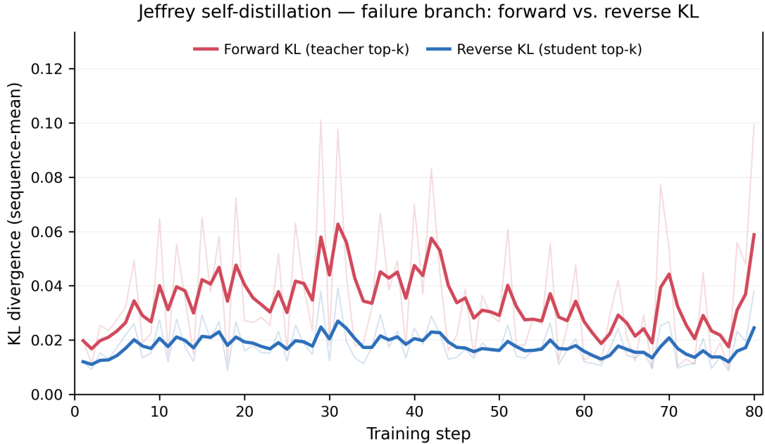
그림 4. 실패 분기에서의 forward KL과 reverse KL 크기 비교
