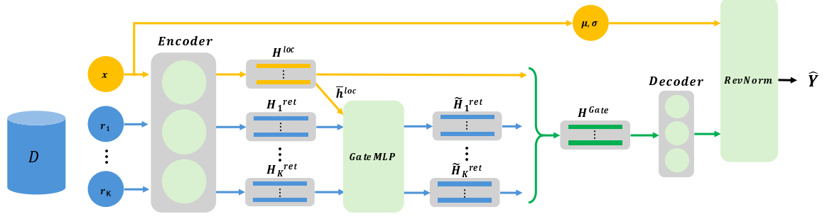
図 2 GateRAF (提案手法) のアーキテクチャ概要
