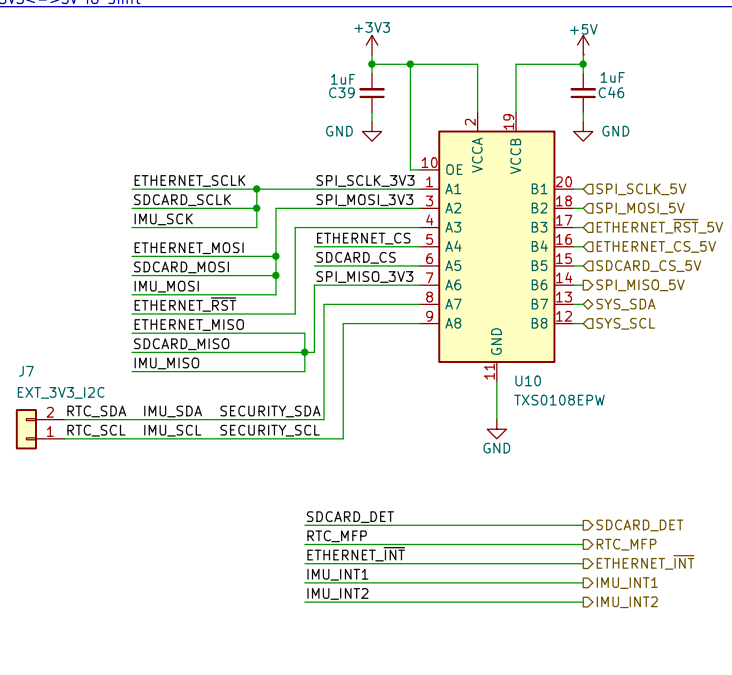
3V3<->5V IO Shift
