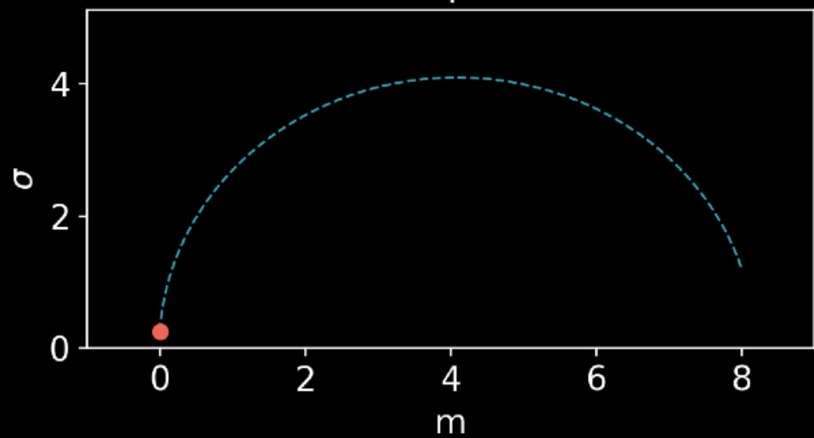
KL Interpolation
