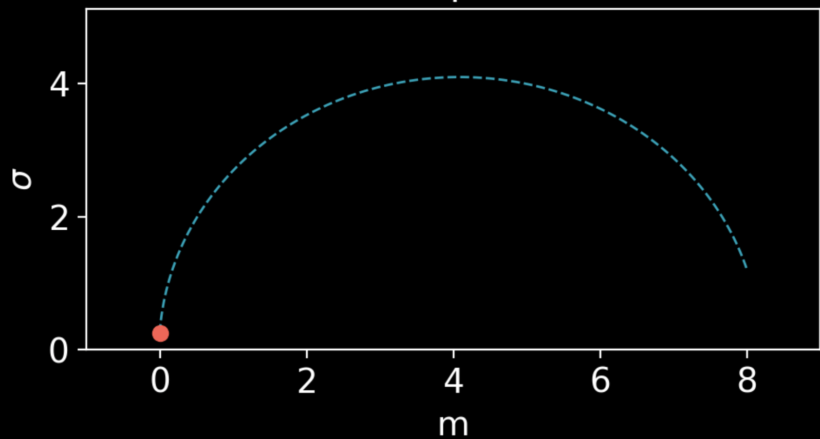
KL Interpolation
