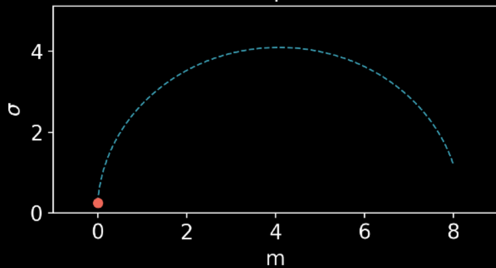
KL Interpolation
