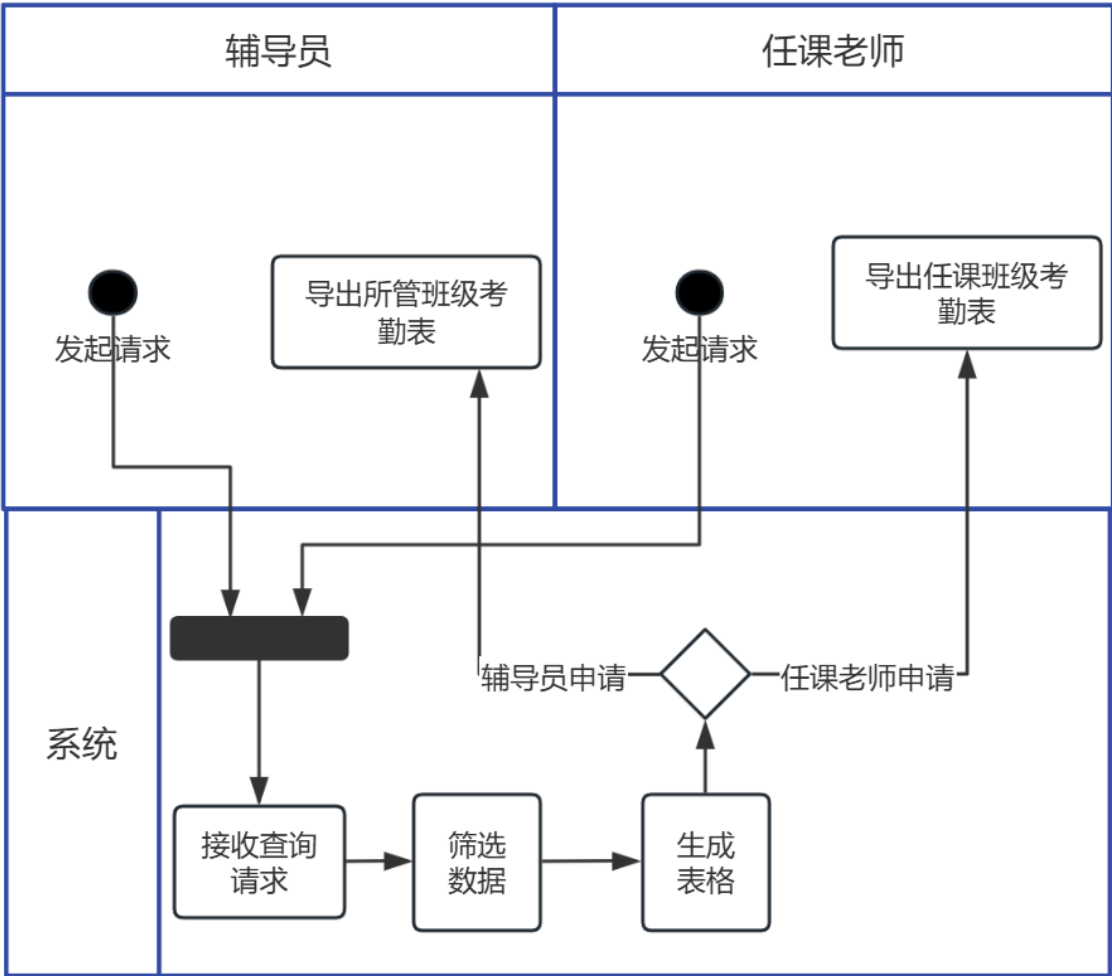
图3-5-3 导出考勤表业务活动图
