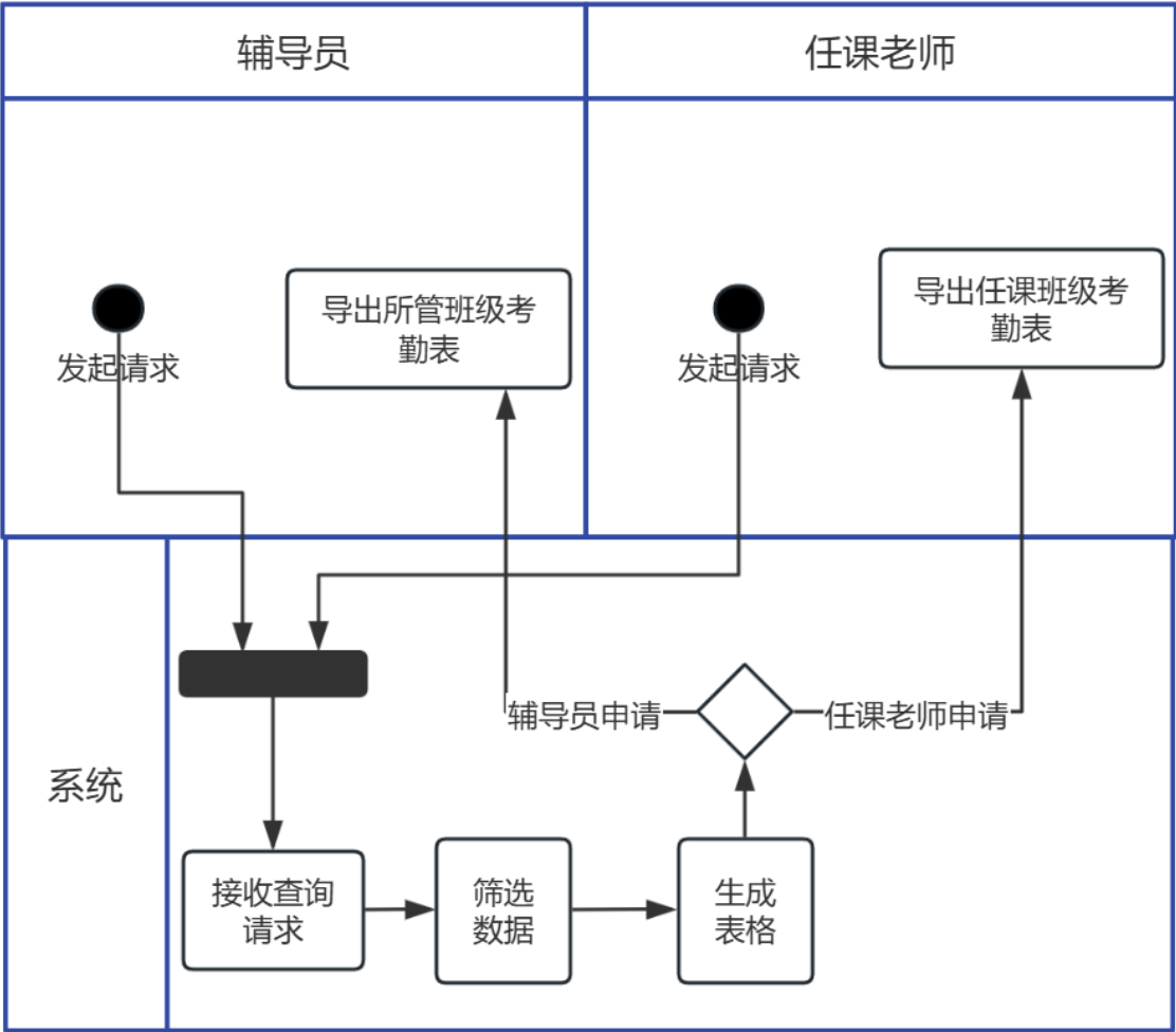
图3-3 导出考勤表业务活动图
