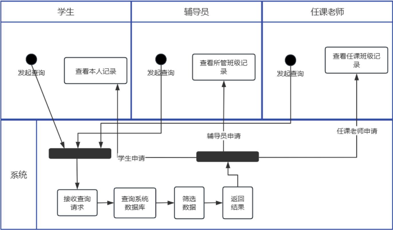
图3-2 查看历史记录活动图
