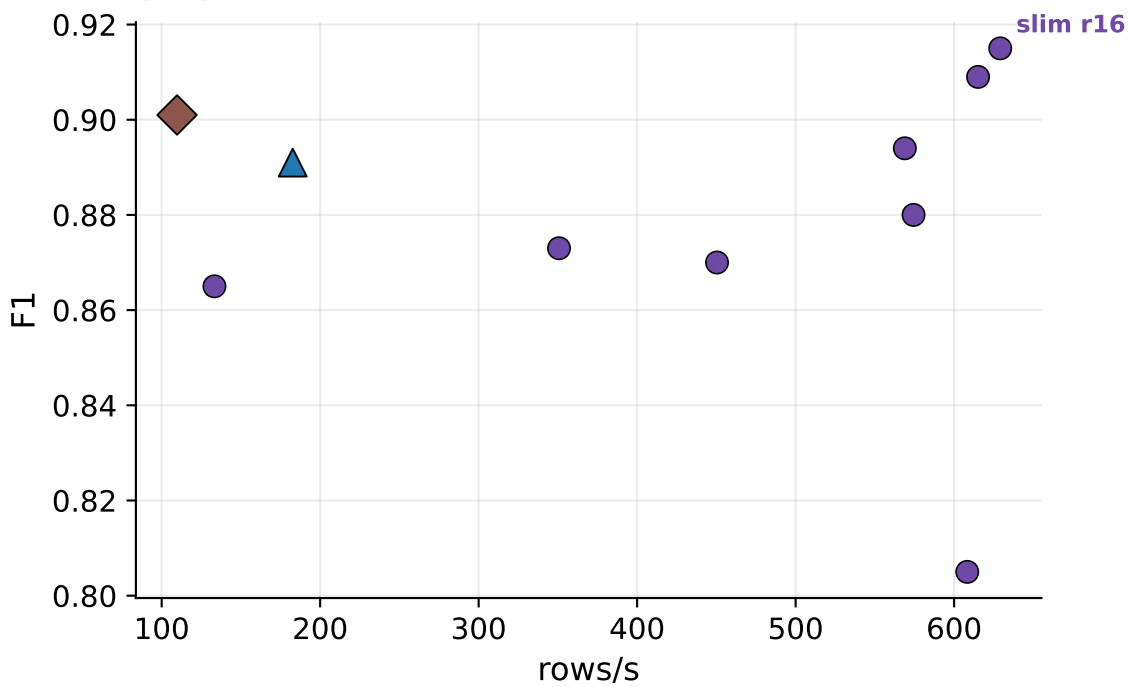
(a2) Llama-3.1-8B — filter
