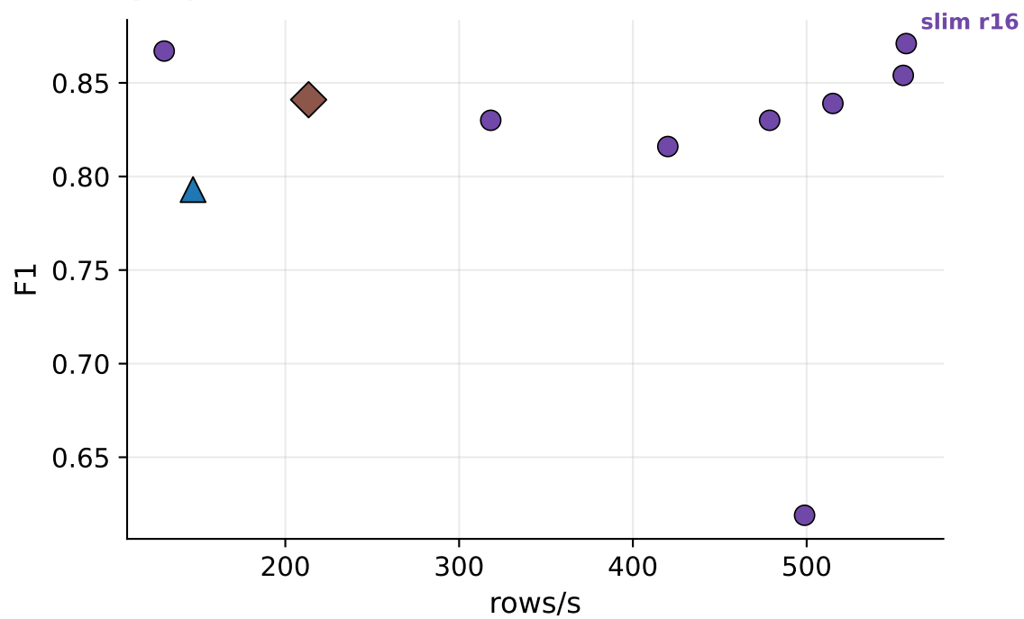
(b2) Llama-3.1-8B — extract
