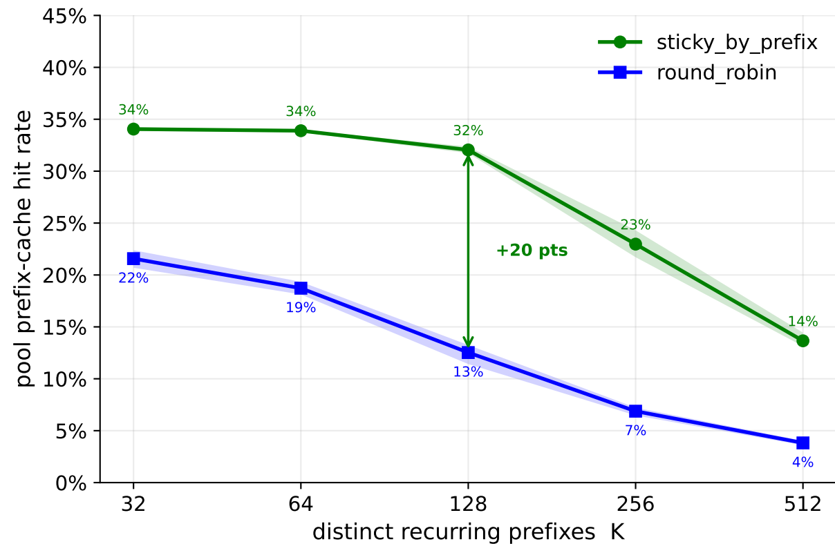
Prefix-cache reuse
