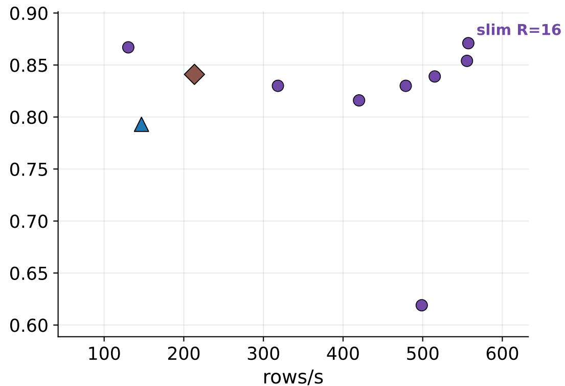
Llama-3.1-8B — extract
