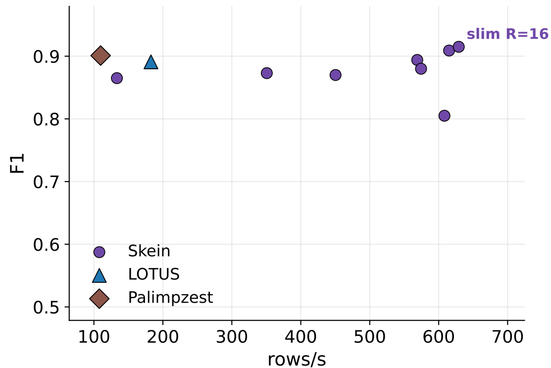
Llama-3.1-8B — filter
