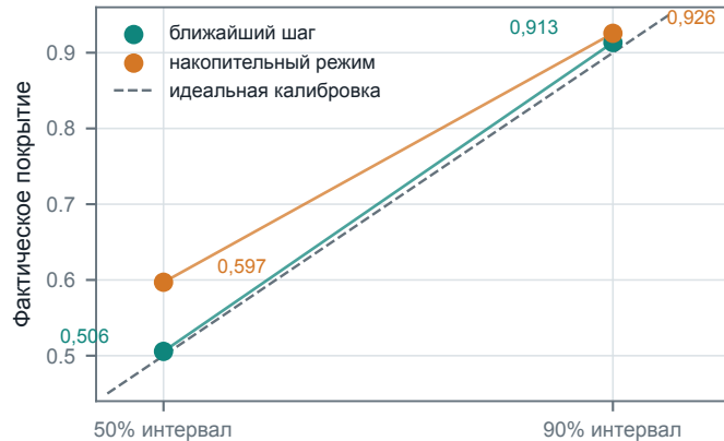
Покрытие интервалов
