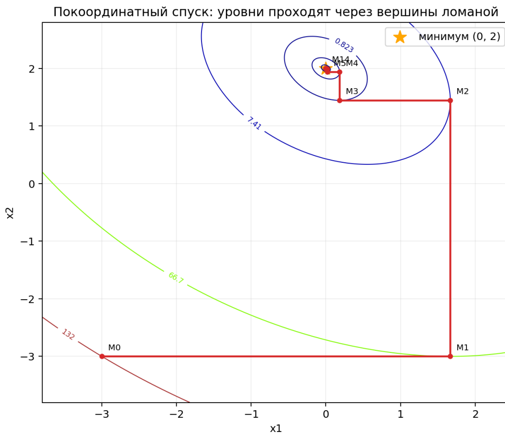
Рис. 4: Покоординатный спуск: ломаная идет параллельно координатным осям.
