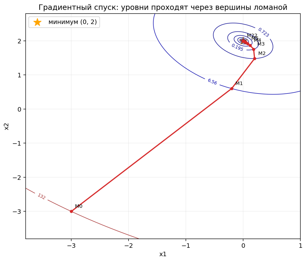
Рис. 5: Градиентный спуск с дроблением шага.
