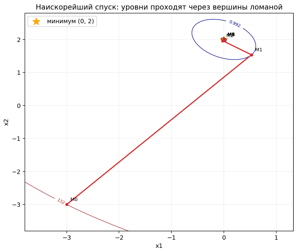
Рис. 6: Наискорейший спуск с точным выбором шага вдоль антиградиента.
