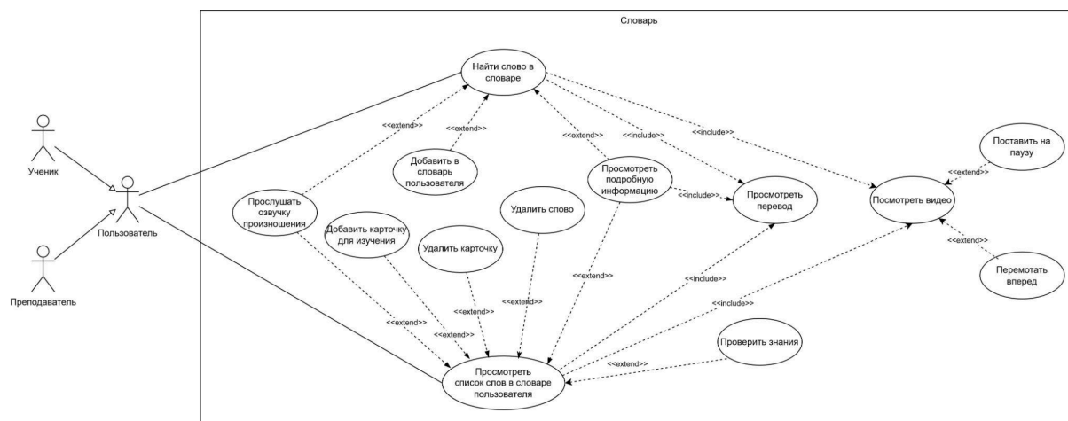
Рисунок 2. Диаграмма Use Case для версии 2.0 веб-приложения Chatty
