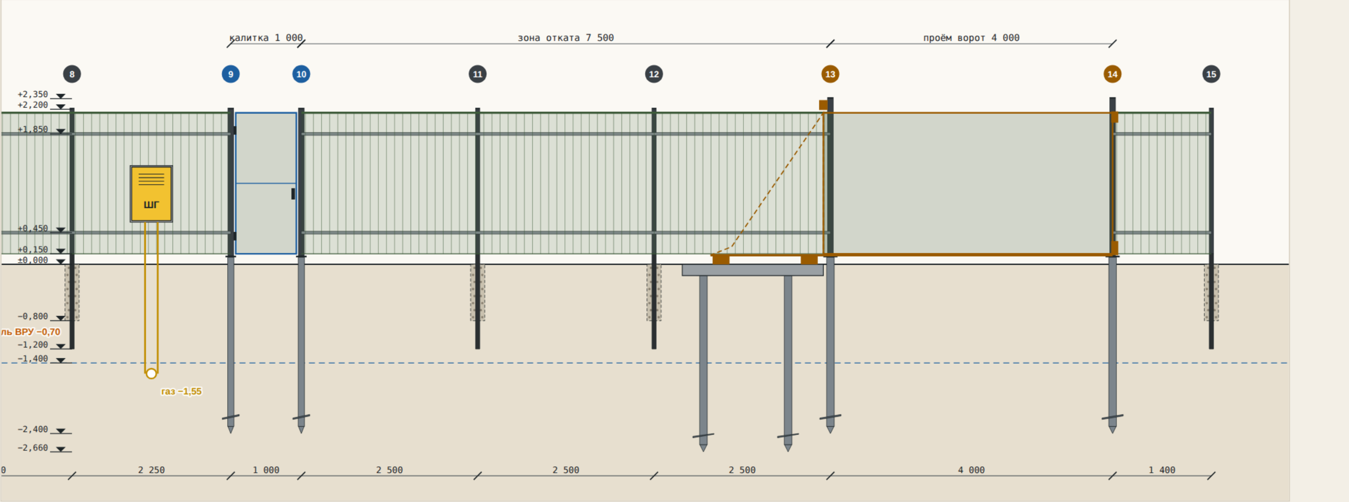
Правая граница — вид снаружи (от соседа справа)
