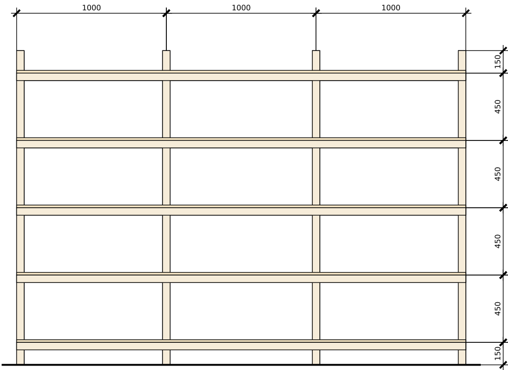
Верстак (поз. 21) — вид спереди М 1:20
