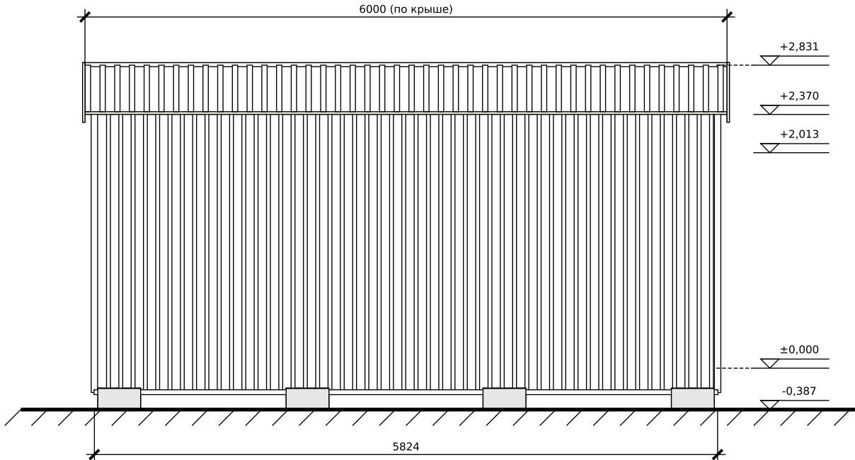
Задний фасад М 1:50
