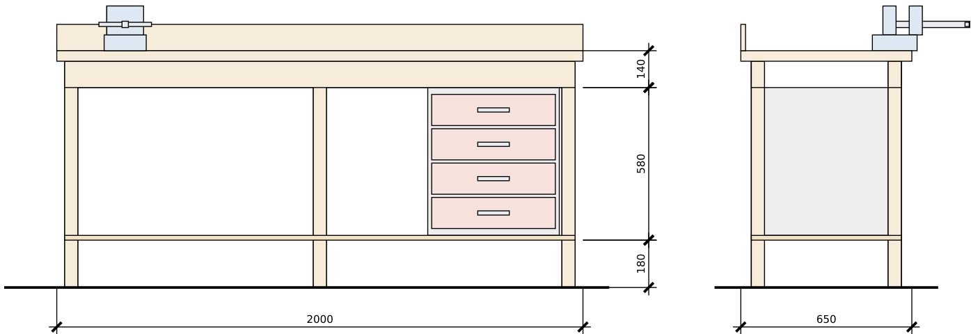
Верстак (поз. 21) — вид спереди М 1:20
