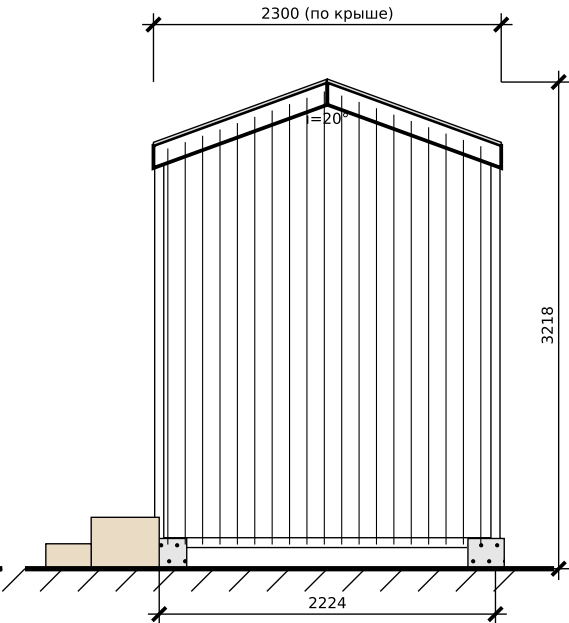
Правый торец М 1:50
