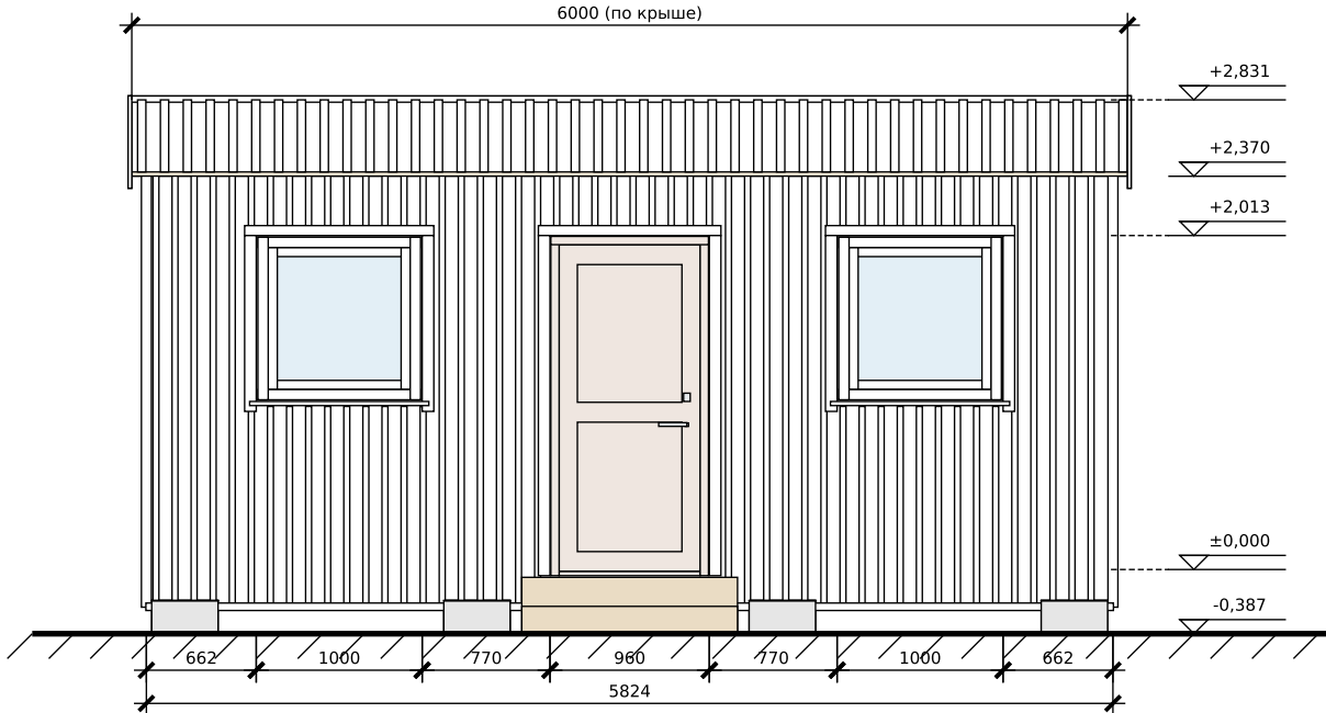
Главный фасад М 1:50
