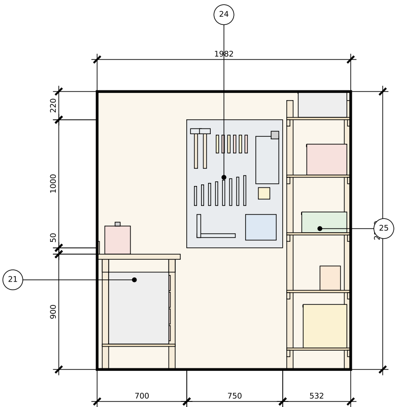
Развёртка В — левый торец М 1:30
