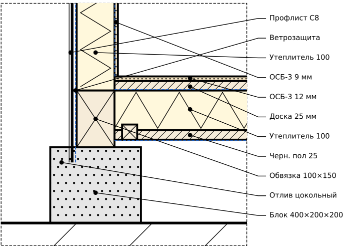
Узел 1 М 1:10
