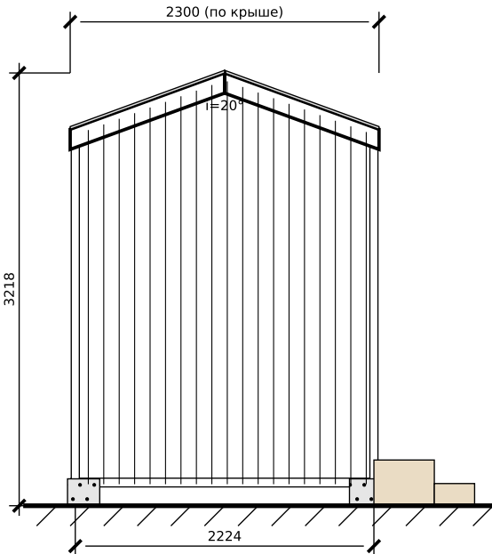
Левый торец М 1:50
