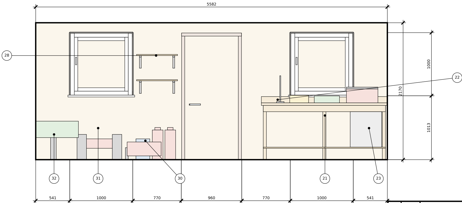
Развёртка Б — стена с дверью и окнами М 1:30
