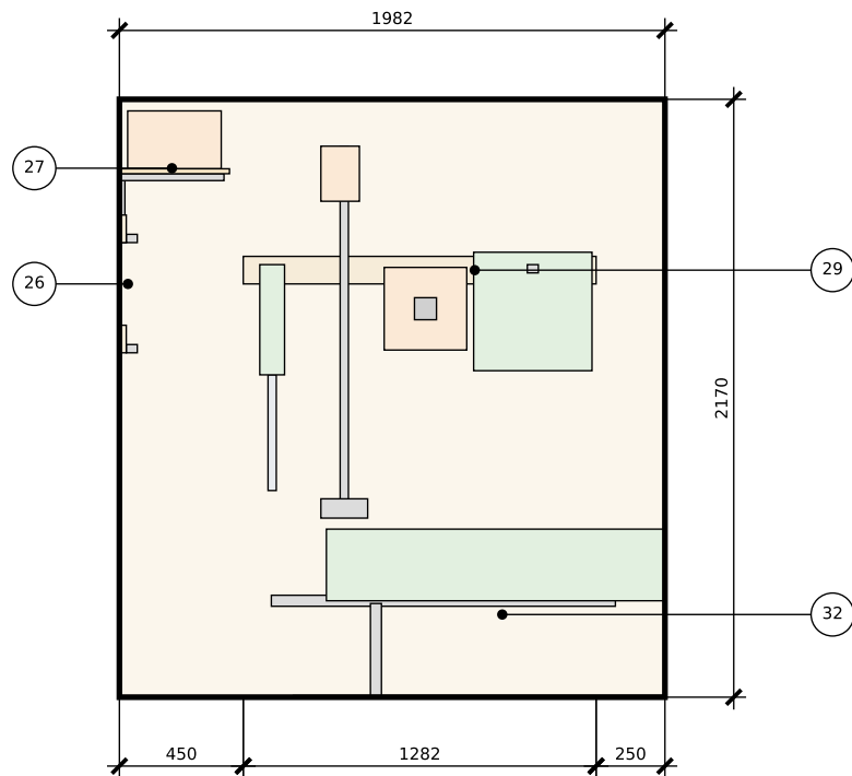
Развёртка Г — правый торец М 1:30
