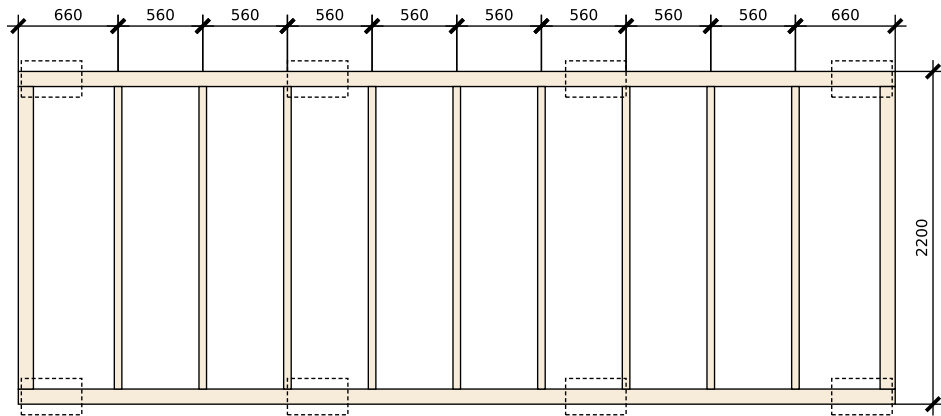
Каркас пола (обвязка, лаги) М 1:50
