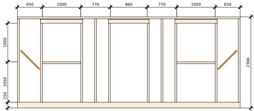
Стена по оси А (с проёмами) М 1:50
