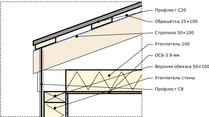
Узел 2 М 1:10
