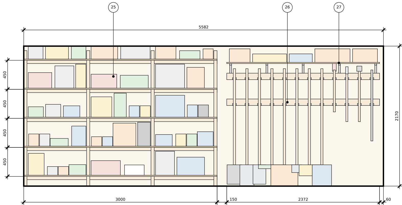
Развёртка А — задняя стена М 1:30
