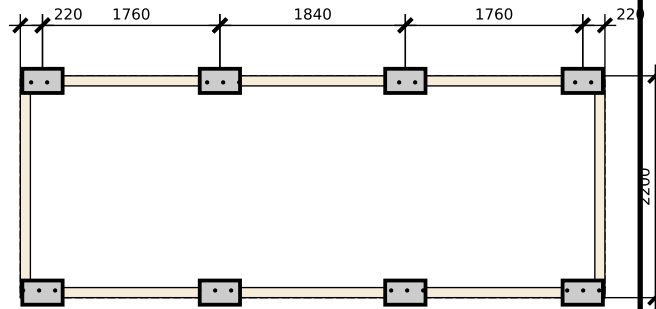
План фундамента М 1:75
