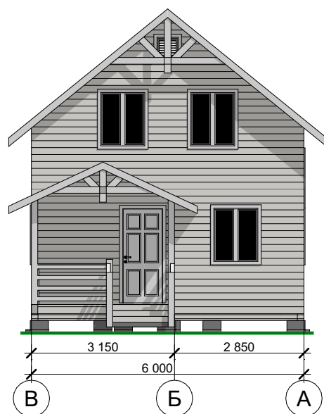
Фасад В-А
