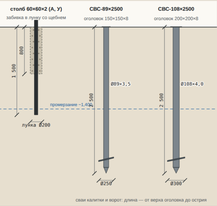
Узел 6 · основания опор
