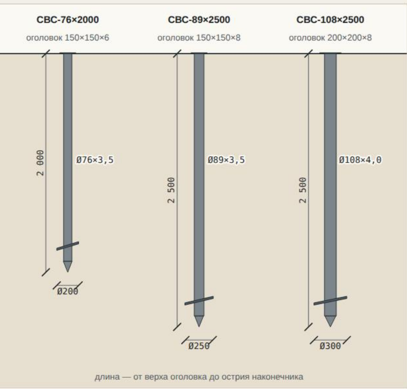
Узел 6 · сваи
