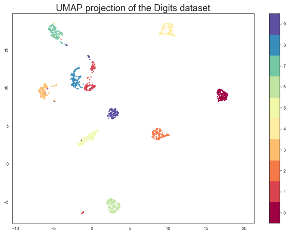
Figura3.17: Proyección UMAP del conjunto de datos Digits . Fuente: documentación de umap-learn, «How to Use UMAP» ( umap-learn.readthedocs.io ). Copyright (c) 2017, Leland McInnes. Licencia BSD de 3 cláusulas.
