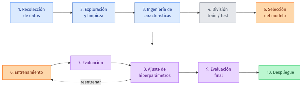
Figura 1.8: El pipeline de Machine Learning: 10 etapas desde la recolección de datos hasta el despliegue.
