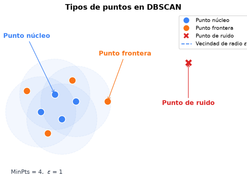
Figura3.6: Clasificación de puntos en DBSCAN: núcleo, frontera y ruido.
