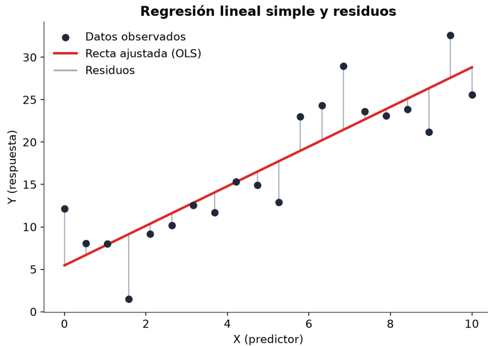
Figura2.1: Regresión lineal simple: recta ajustada y residuos.
