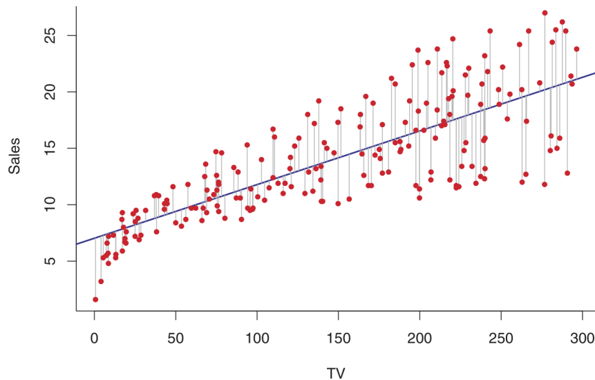
Figura2.2: Ajuste por mínimos cuadrados de Sales sobre TV en el conjunto de datos Advertising . Fuente: James, G., Witten, D., Hastie, T., & Tibshirani, R. (2013). An Introduction to Statistical Learning , Figura 3.1. Springer. Libro de libre distribución para uso educativo ( statlearning.com ).
