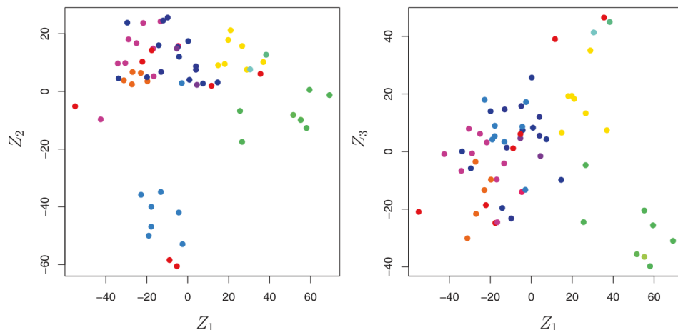
Figura 3.13: Proyección de las líneas celulares de cáncer NCI60 (6830 genes) sobre sus tres primeras componentes principales. Fuente: James, G., Witten, D., Hastie, T., & Tibshirani, R. (2013). An Introduction to Statistical Learning , Figura 10.15. Springer. Libro de libre distribución para uso educativo ( statlearning.com ).
