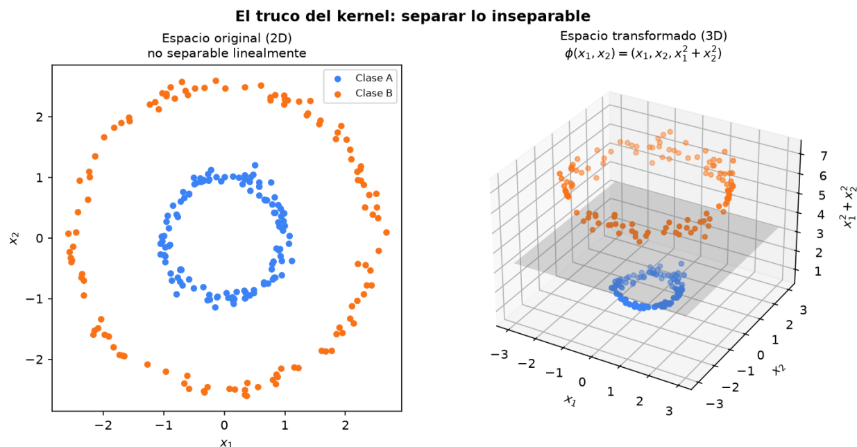
Figura 3.15: El truco del kernel : datos no separables en 2D se vuelven separables al proyectarlos a una dimensión adicional.
