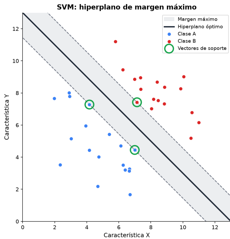
Figura2.10: SVM: hiperplano de margen máximo y vectores de soporte.
