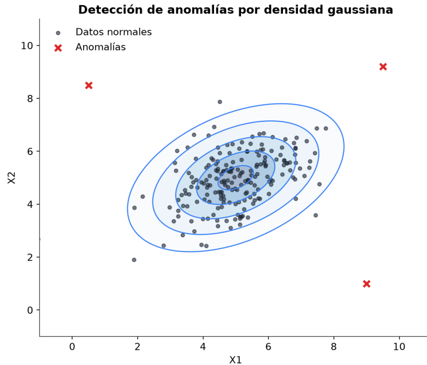
Figura 3.19: Detección de anomalías mediante estimación de densidad gaussiana.
