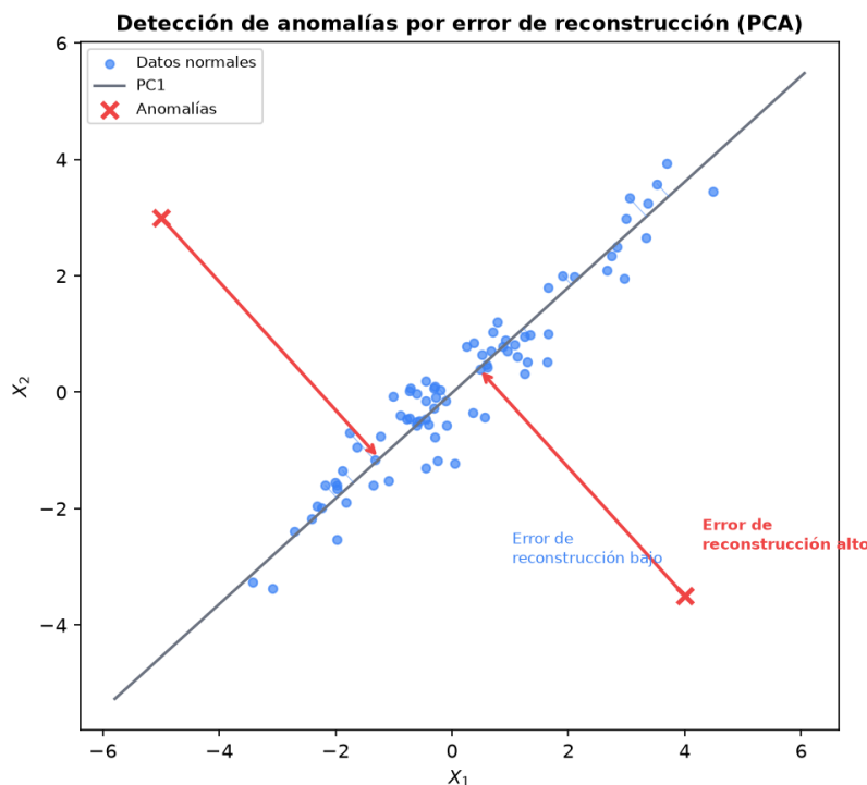
Figura 3.20: Detección de anomalías mediante el error de reconstrucción de PCA.
