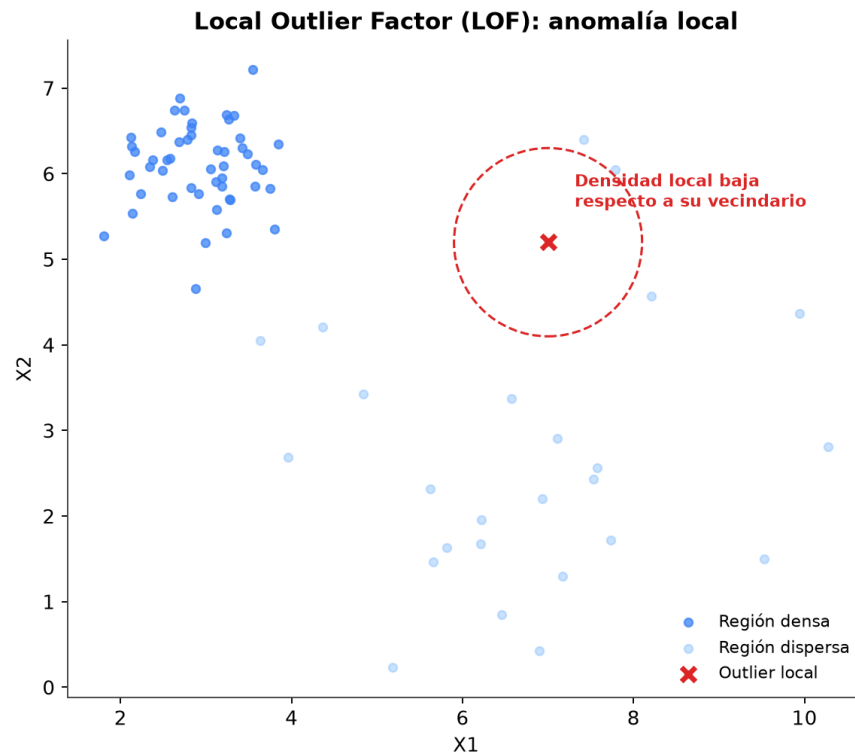
Figura3.22: Local Outlier Factor : una anomalía local no destaca en un análisis global.
