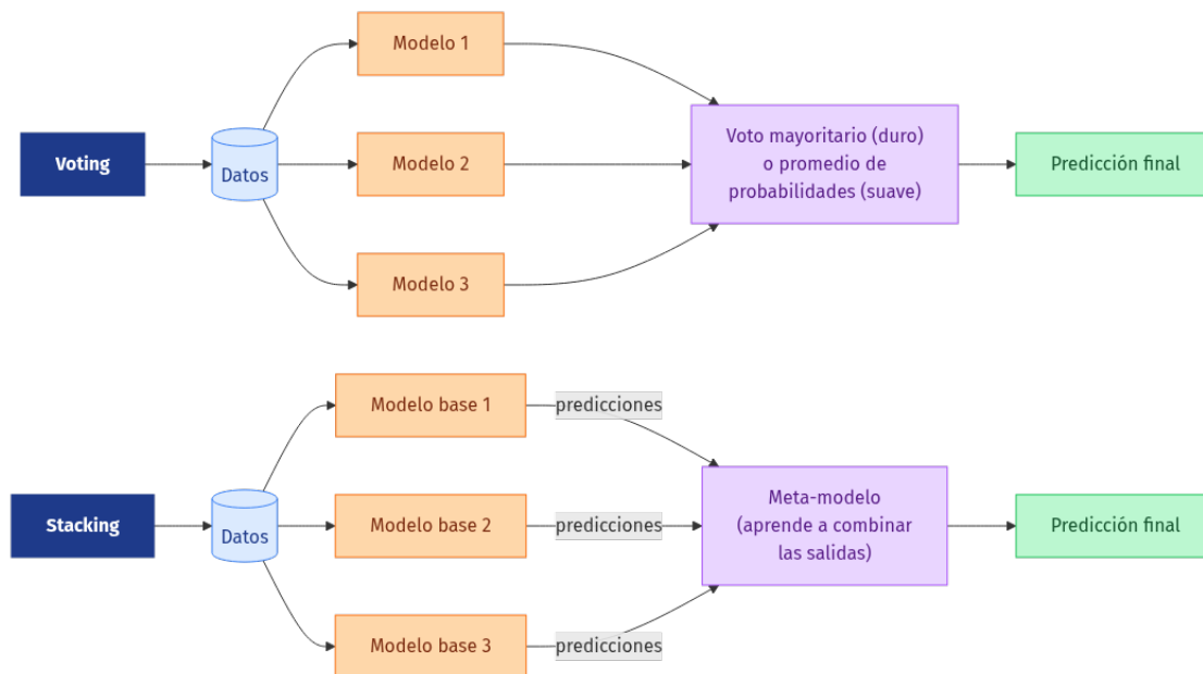
Figura2.11: Voting frente a stacking : regla fija de combinación frente a meta-modelo que aprende a combinar.
