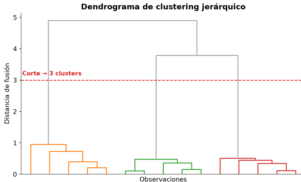
Figura 3.4: Dendrograma de clustering jerárquico con un corte que produce 3 clusters.
