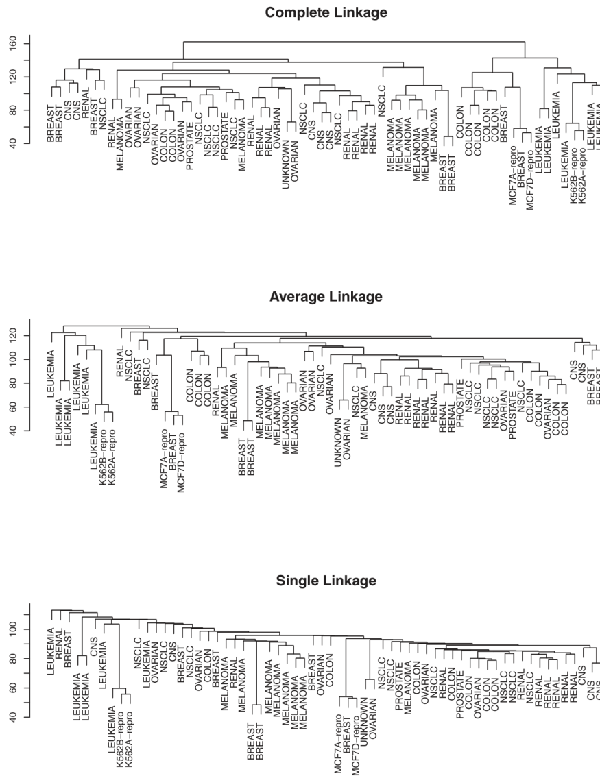
Figura3.5: Clustering jerárquico del conjunto de datos NCI60 con enlace completo, promedio y simple. Fuente: James, G., Witten, D., Hastie, T., & Tibshirani, R. (2013). An Introduction to Statistical Learning , Figura 10.17. Springer. Libro de libre distribución para uso educativo ( statlearning.com ).
