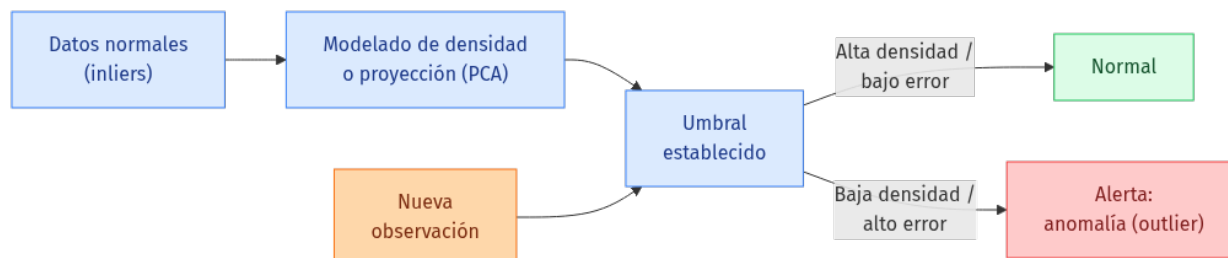
Figura 3.18: Esquema general de los enfoques estadísticos y de reconstrucción: modelar lo normal, fijar un umbral y marcar lo que queda fuera.
