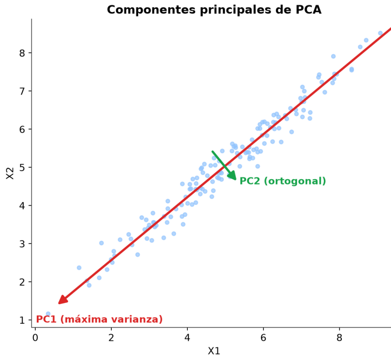
Figura 3.12: Componentes principales: PC1 captura la máxima varianza, PC2 es ortogonal.
