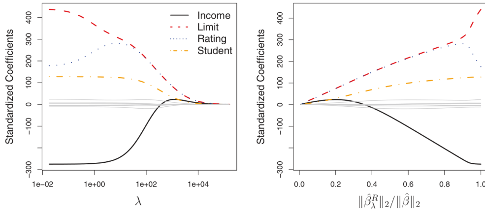
Figura 2.5: Coeficientes de regresión Ridge estandarizados para el conjunto de datos Credit . Fuente: James, G., Witten, D., Hastie, T., & Tibshirani, R. (2013). An Introduction to Statistical Learning , Figura 6.4. Springer. Libro de libre distribución para uso educativo ( statlearning.com ).
