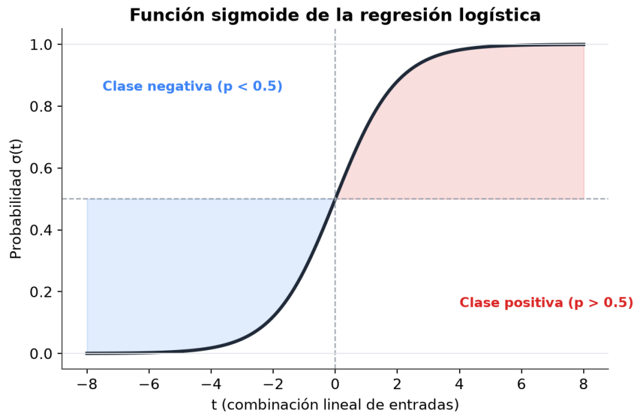
Figura2.6: Función sigmoide de la regresión logística.
