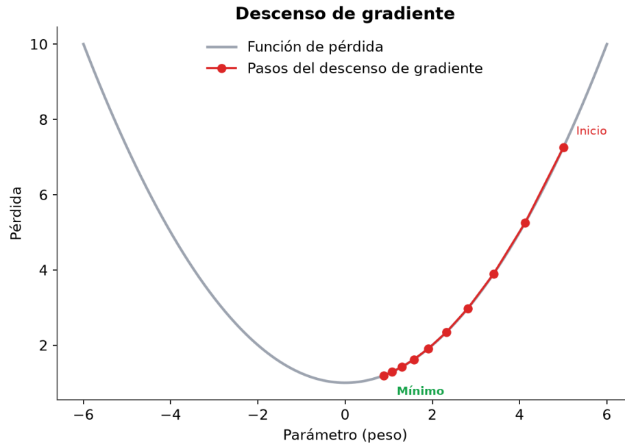
Figura2.3: Descenso de gradiente: pasos iterativos hacia el mínimo de la pérdida.
