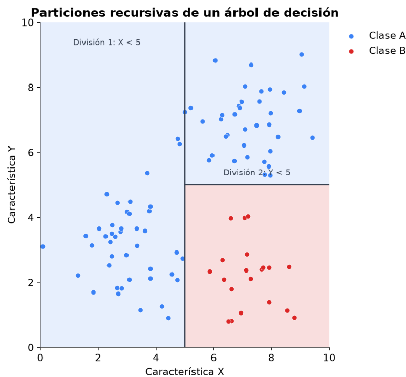
Figura2.8: Particiones recursivas de un árbol de decisión sobre dos características.
