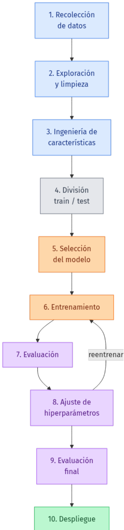
Figura3.4: El pipeline de Machine Learning : 10 etapas desde la recolección de datos hasta el despliegue.
