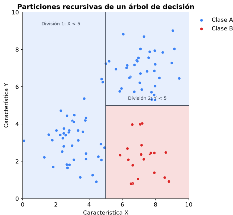
Figura6.3: Particiones recursivas de un árbol de decisión sobre dos características.
