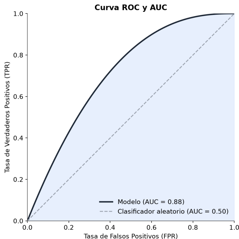
Figura 6.8: Curva ROC y área bajo la curva (AUC).
