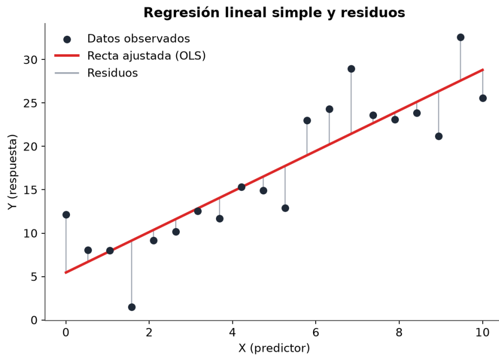
Figura5.1: Regresión lineal simple: recta ajustada y residuos.
