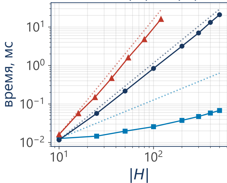
(а) сложность: O(|H|)/O(|H|^2)/O(|H|^3)
