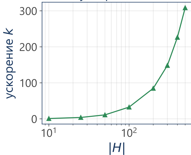
(б) ускорение Алг.2
