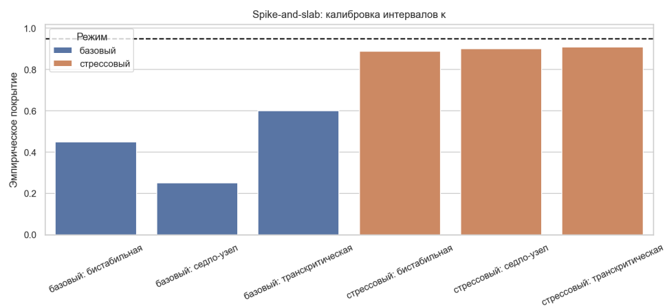
Рисунок 3 - Эмпирическое покрытие 95%-го интервала Bayesian SINDy для скорости восстановления
