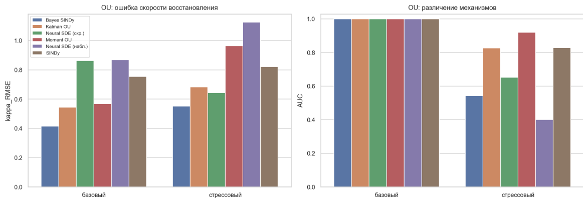
Рисунок 1 - Результаты OU-эксперимента при одинаковом горизонте
