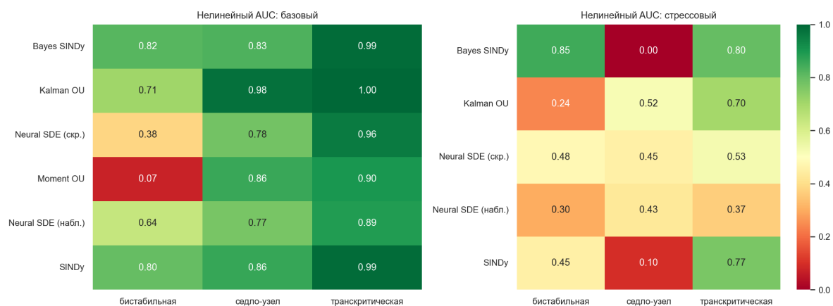
Рисунок 2 - AUC по трем нормальным формам при одинаковой траектории локальной устойчивости
