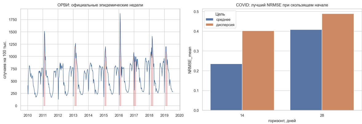
Рисунок 4 - Слева — размеченный недельный ряд ОРВИ; справа — прогноз COVID-индикаторов со скользящим началом на одинаковых датах отсечения
