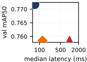
NEU · YOLOv8n
