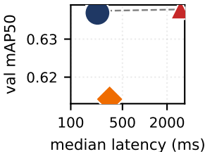
GC10 · YOLOv8s
