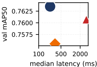
NEU · YOLOv8s
