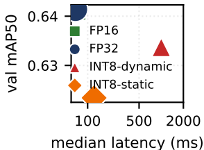
GC10 · YOLOv8n
