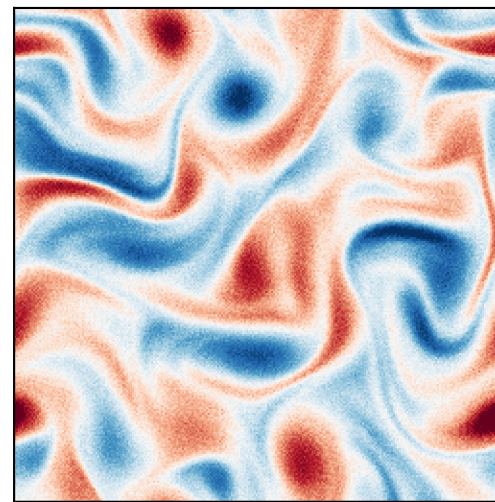
DDIM step 40
