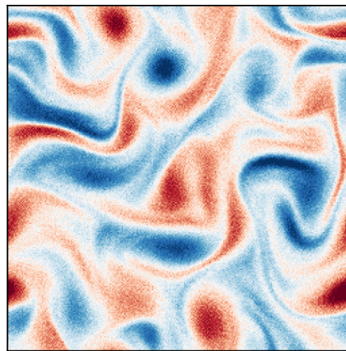
DDIM step 20
