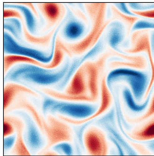
DDIM step 80
