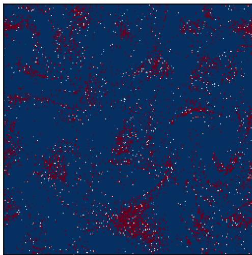
DDIM step 1
