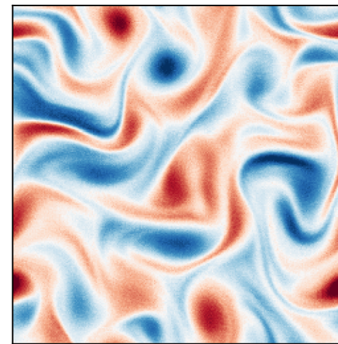
DDIM step 100
