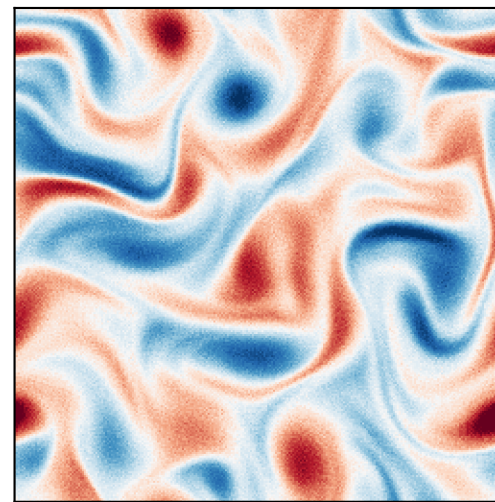
DDIM step 60
