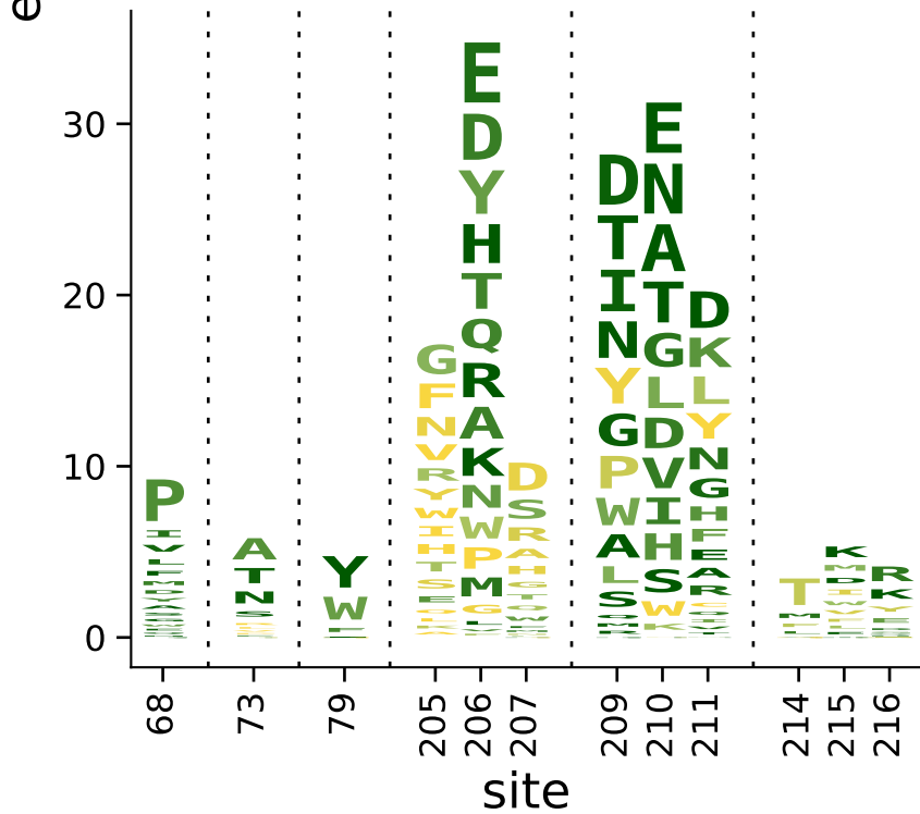
RSM01-Fab
