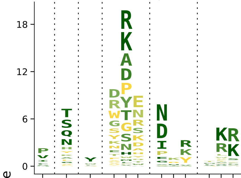
RSM01-IgG
