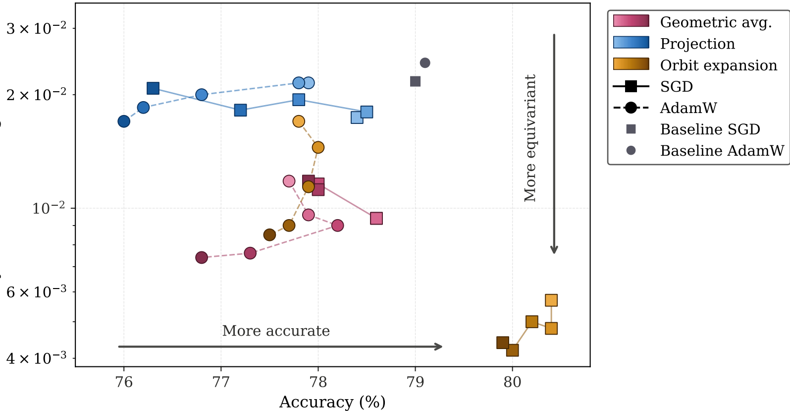
Symmetric KL divergence
