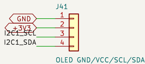
OLED GND/VCC/SCL/SDA
