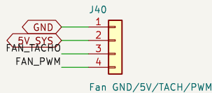
Fan GND/5V/TACH/PWM
