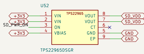
TPS22965DSGR
