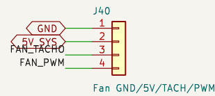
Fan GND/5V/TACH/PWM
