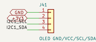
OLED GND/VCC/SCL/SDA
