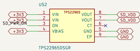
TPS22965DSGR
