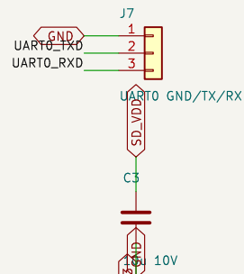
UART0 GND/TX/RX
