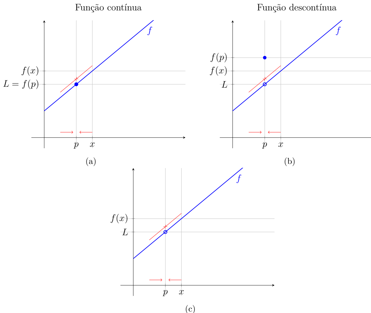
Figura 27: Comparação entre os limites ( L ) das funções: em (a), uma função contínua em p e L = f(p) . Em (b), uma função descontínua em p , com f(p) \neq L . Em (c), a função f tende a L , ainda que p não esteja no domínio.
