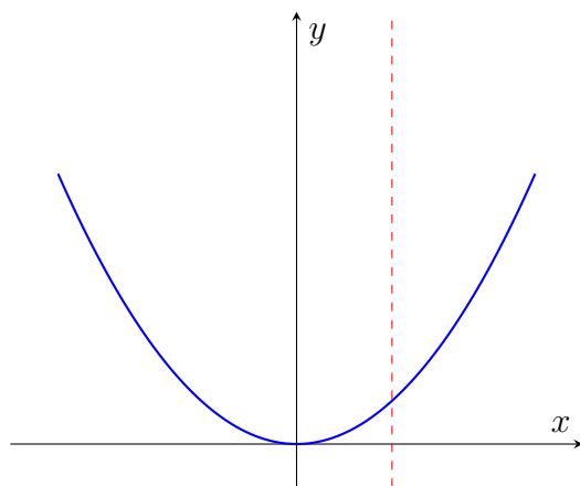
(a) Cada valor de x tem um único valor de y .
