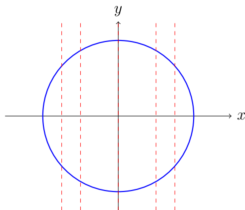
(b) Alguns valores de x têm dois valores de y .
