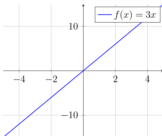
Figura 12: Função afim f(x) = 3x
