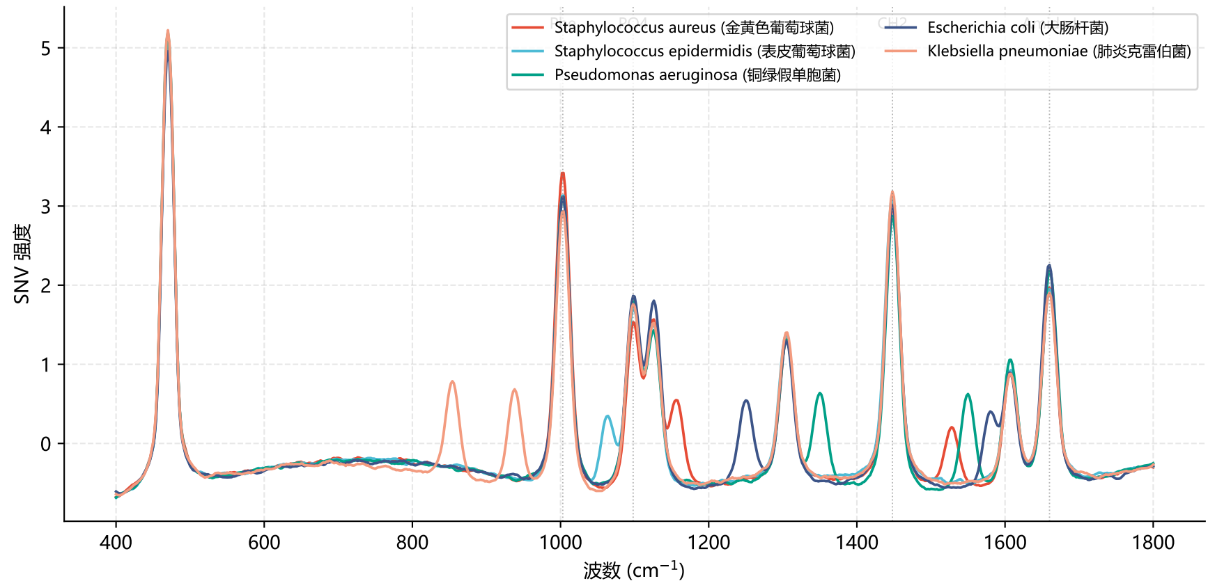
预处理后 5 类菌种平均光谱对比
