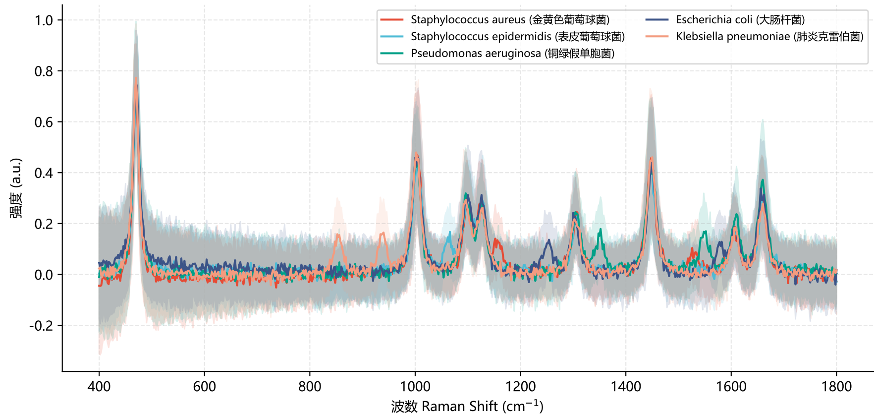
原始拉曼光谱概览 (每类均值 \pm 标准差)
