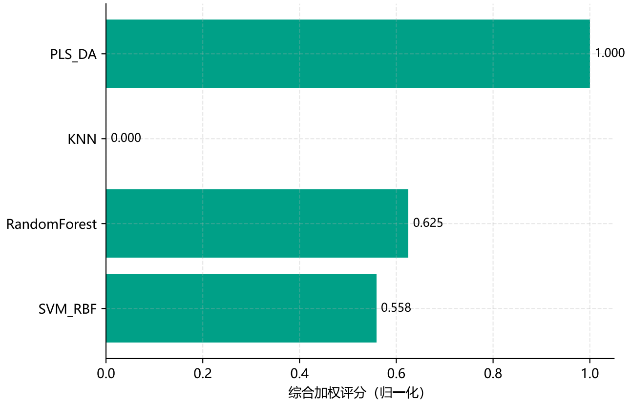
三维度加权综合评分 (0.4•Acc + 0.4•F1 + 0.2•速度)
