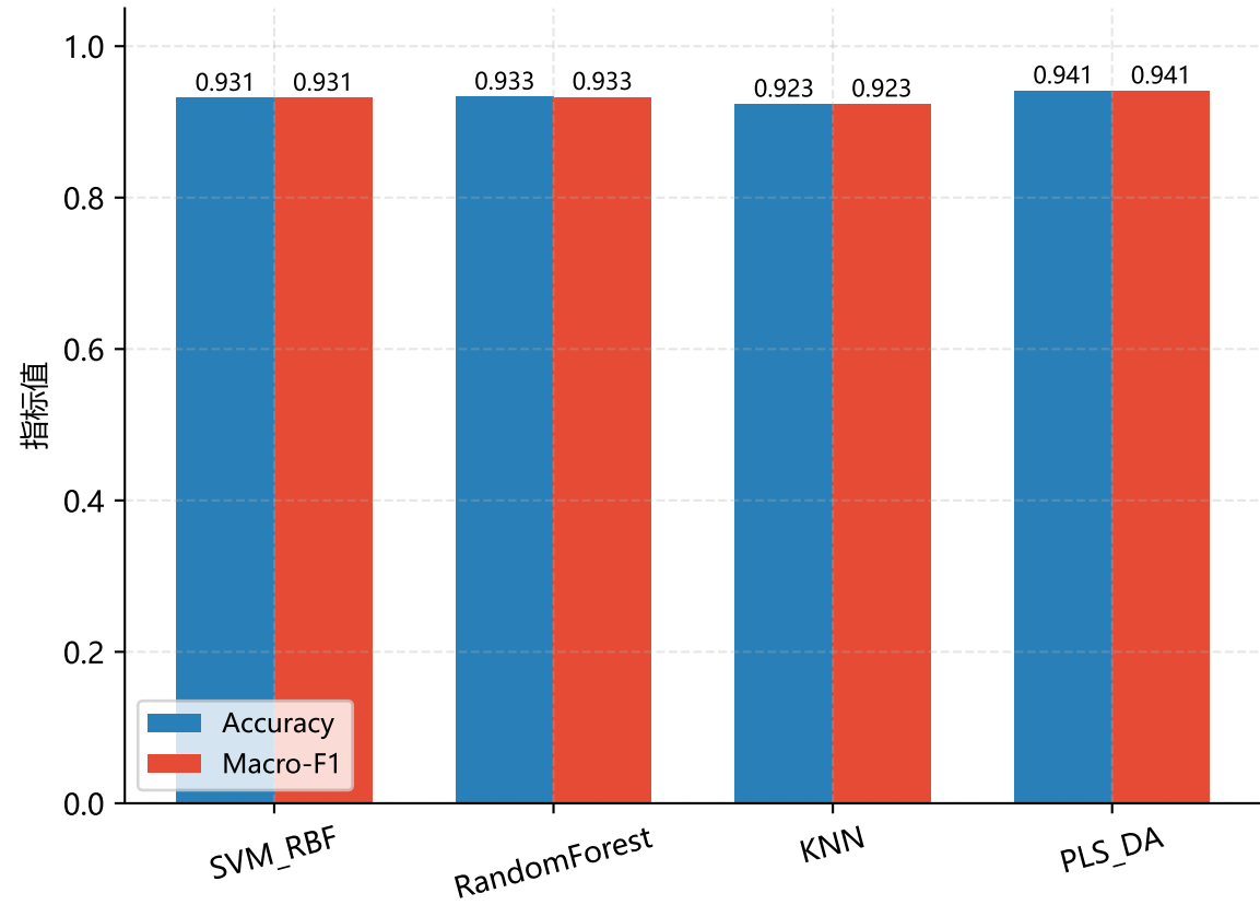
分类模型: Accuracy & Macro-F1
