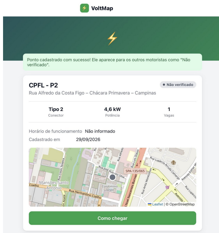
Figura 6 – Página de detalhes de um ponto de recarga
