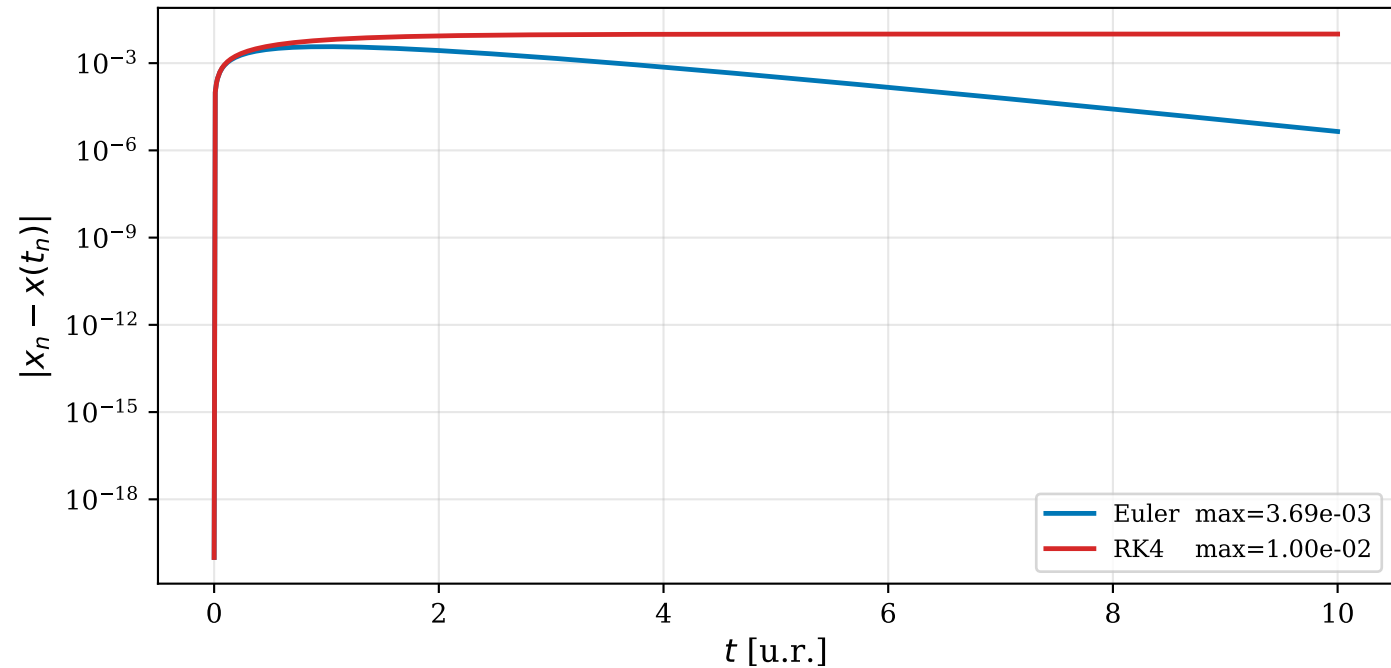
Error absoluto en posición — \Delta t = 0.01
