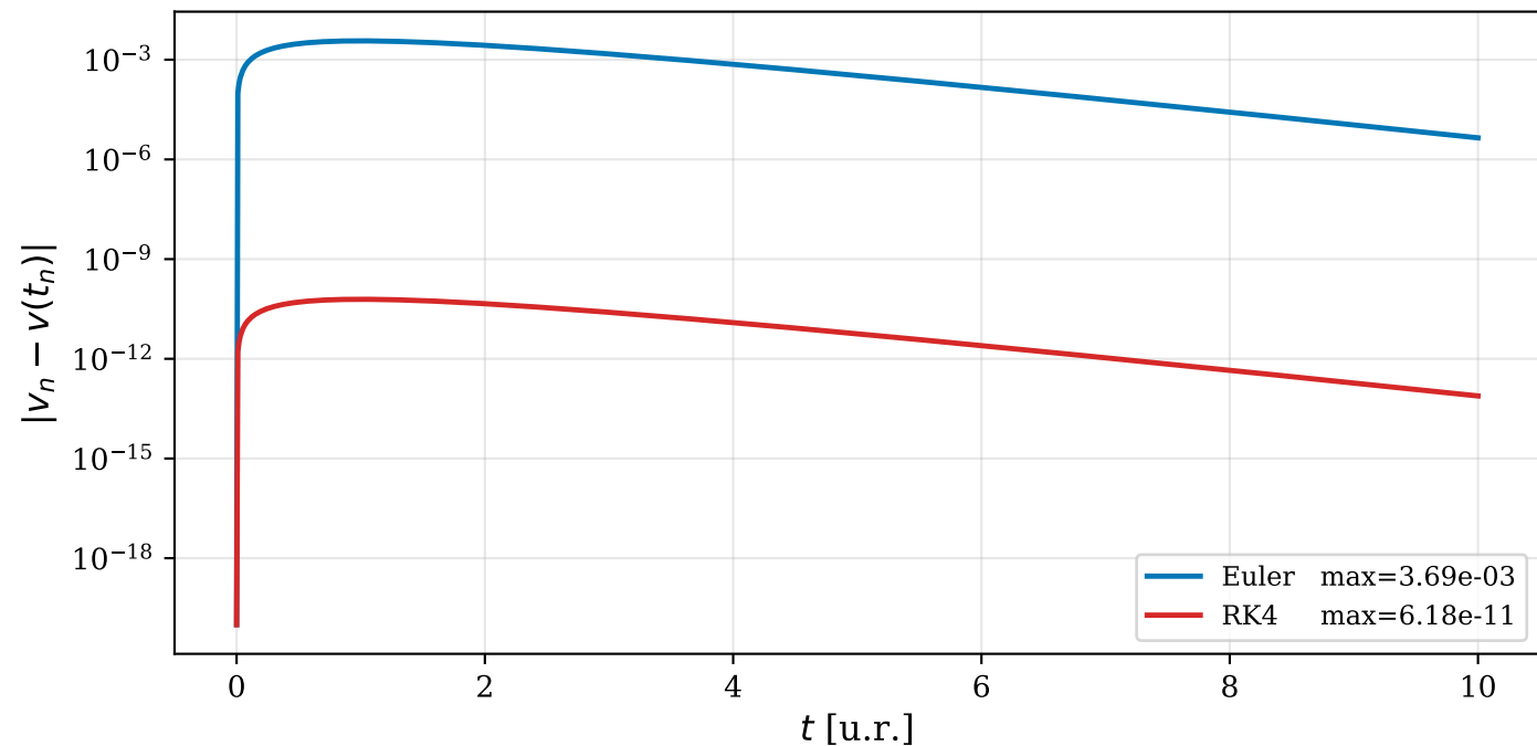
Error absoluto en velocidad — \Delta t = 0.01
