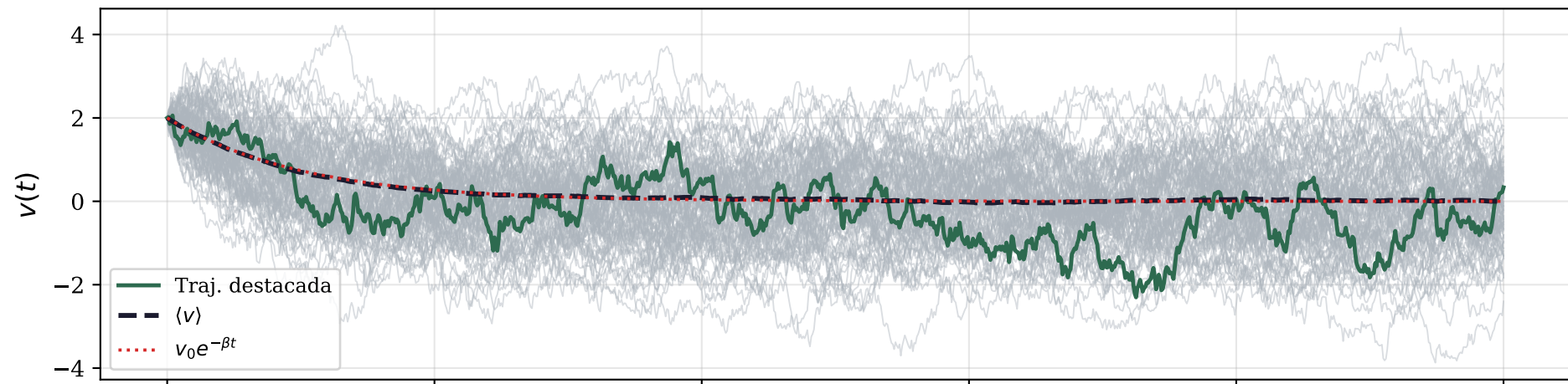
Trayectorias Brownianas — Euler-Maruyama ( N = 2000 , \Delta t = 0.01 )
