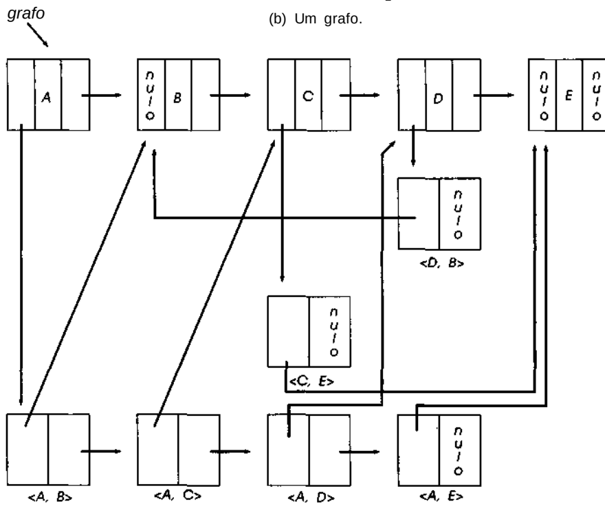
Figura 8.3.1 Representação ligada de um grafo.
