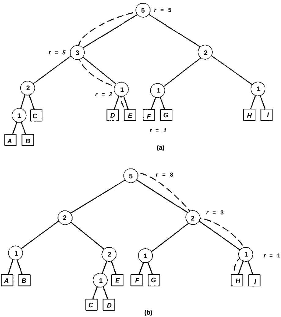
Figura 5.4.2 Localizando o n ésimo elemento de uma lista representada por árvore.
