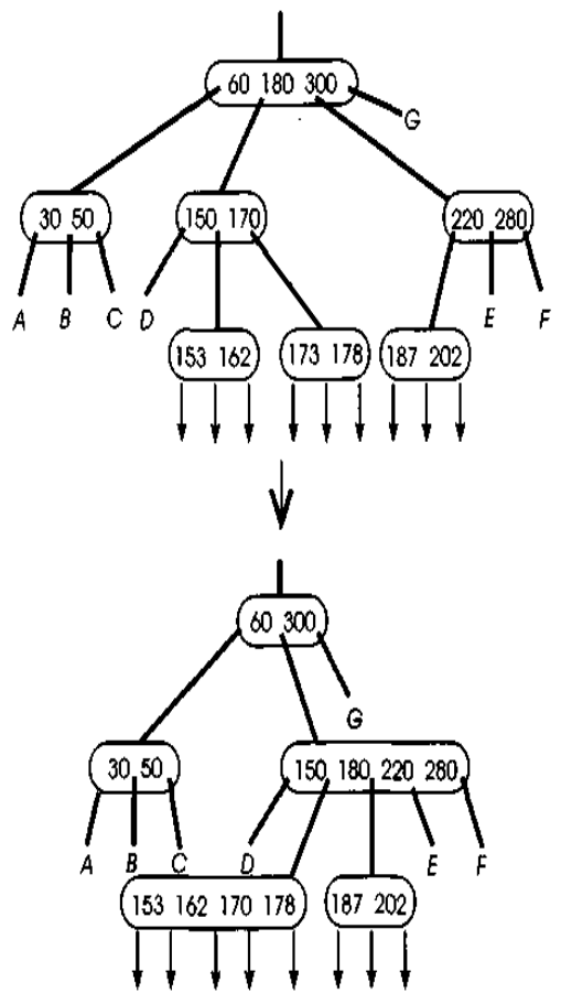
(b) Eliminando 173, uma consolidação dupla
