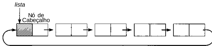
Figura 4.5.3 Uma lista circular com um nó de cabeçalho.
