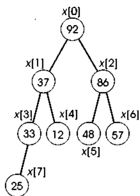
(a) Árvore original.
