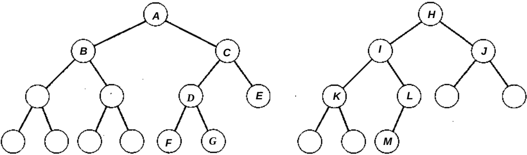
(b) Extensões quase completas
