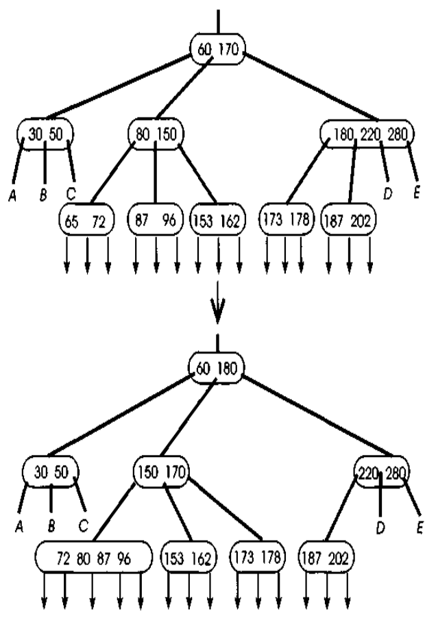
(a) Eliminando 65, consolidando e emprestando
