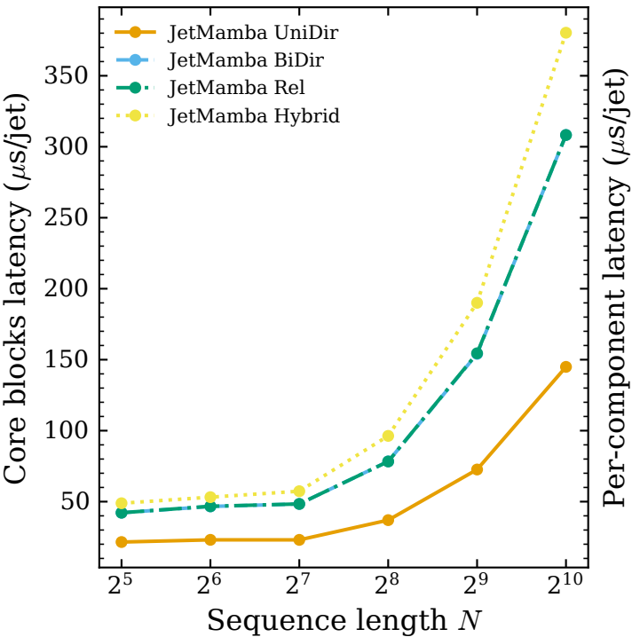
JetMamba: SSM blocks
