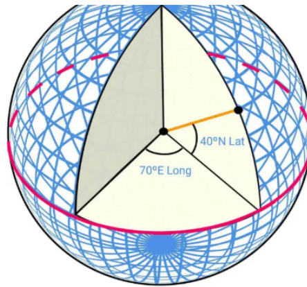
Figure 1 Latitude and Longitude (source: [5])
