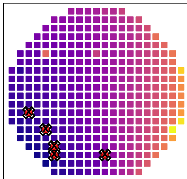
LHS
