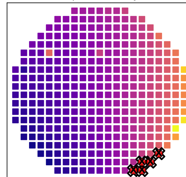
Top5Similarity
