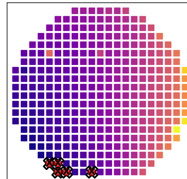
ODAL
