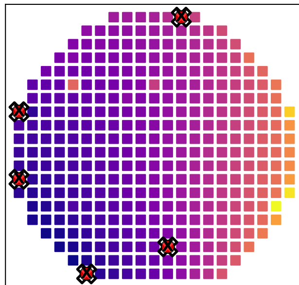
Farthest
