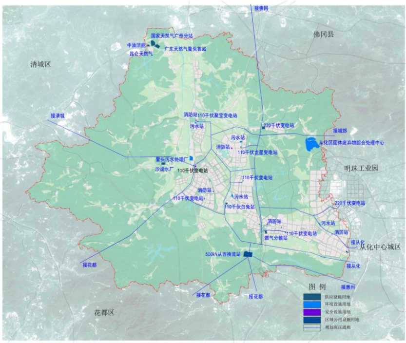
图 7 鳌头镇重大基础设施空间布局图
