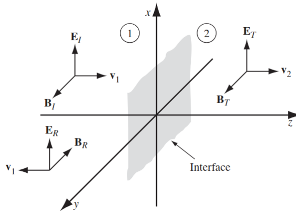
120. ábra. Elektromágneses hullám határfelületen
