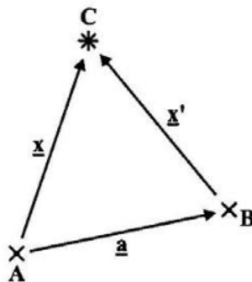
296. ábra. Homogén univerzum két megfigyelővel és egy csillaggal.
