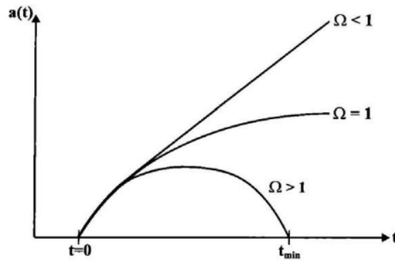
298. ábra. Az univerzum sorsa az \Omega paraméter függvényében. Ha \Omega < 1 , akkor az univerzum nyílt, ha \Omega = 1 , akkor lapos, ha \Omega > 1 , akkor zárt geometriájú.
