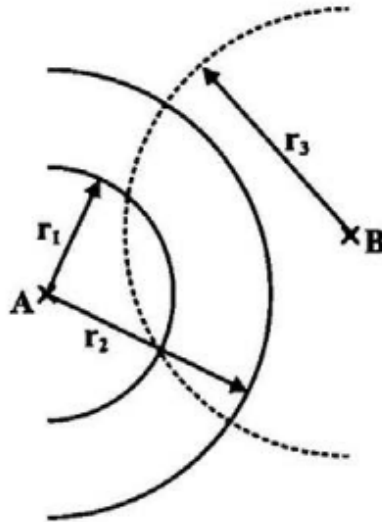
295. ábra. A Kopernikuszi elv szemléltetése. Ha az univerzum bármelyik pontból izotróp és a kopernikuszi elv igaz, akkor homogen is kell legyen.
