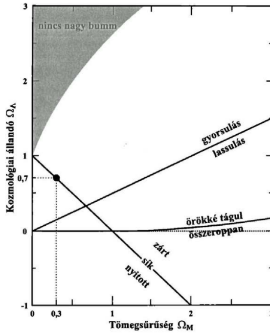
301. ábra. Az univerzum tágulásának időfejlődése különböző kozmológiai paraméterek mellett.
