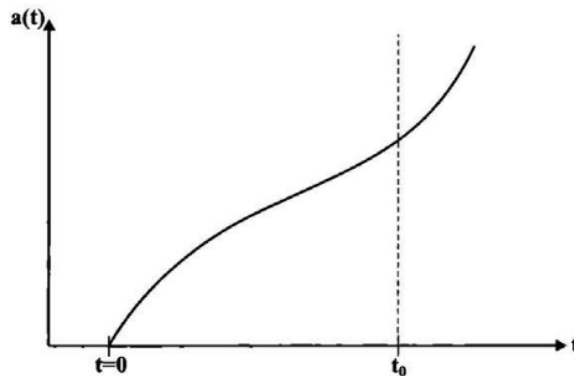
300. ábra. Az univerzum tágulási paraméterének időfejlődése jelenlegi tudásunk szerint.
