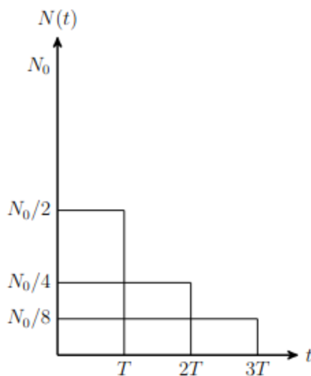
214. ábra. Exponenciális bomlástörvény.
