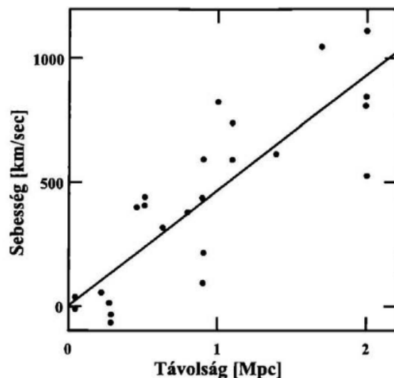
303. ábra. A távolodási sebesség és a luminozitási távolság kapcsolatát feltáró Hubble-diagram. A pontokra illesztett egyenes a Hubble-törvény, annak meredeksége a Hubble-állandó.
