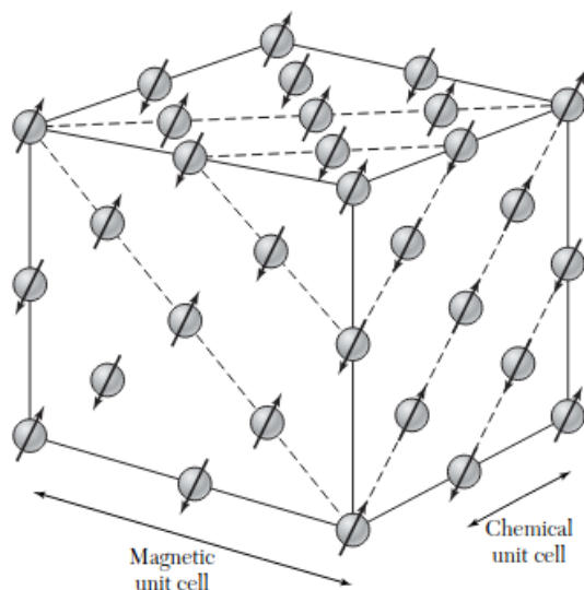
258. ábra. Antiferromágneses anyag illusztrációja.
