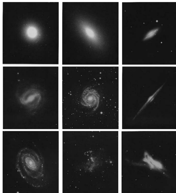
308. ábra. Néhány példa a különböző galaxis osztályokra. Jobbról-balra és fentről-lefelé haladva: NGC 4278 (E1), NGC 3377 (E6), NGC 5866 (S0), NGC 175 (SBa), NGC 6814 (Sb), NGC 4565 (Sb, szélével), NGCX 5364 (Sc), Ho II (Irr I), NGC 520 (Irr II).
