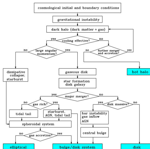
307. ábra. A galaxisok kialakulásának "flowchart"-ja. Ez a diagram bemutatja, hogy a különböző tulajdonságok hogyan kapcsolódnak egymáshoz és hogyan befolyásolják a galaxis fejlődését.
