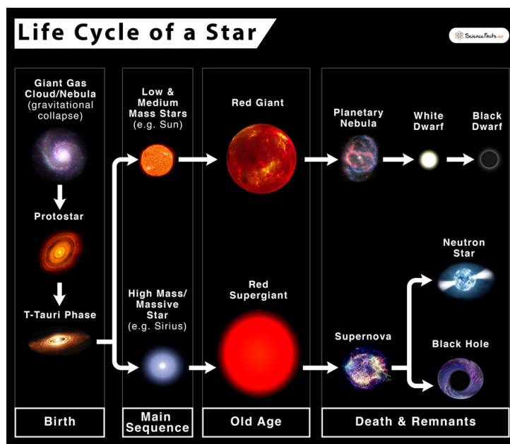
310. ábra. Különböző tömegű csillagok lehetséges evolúciója.
