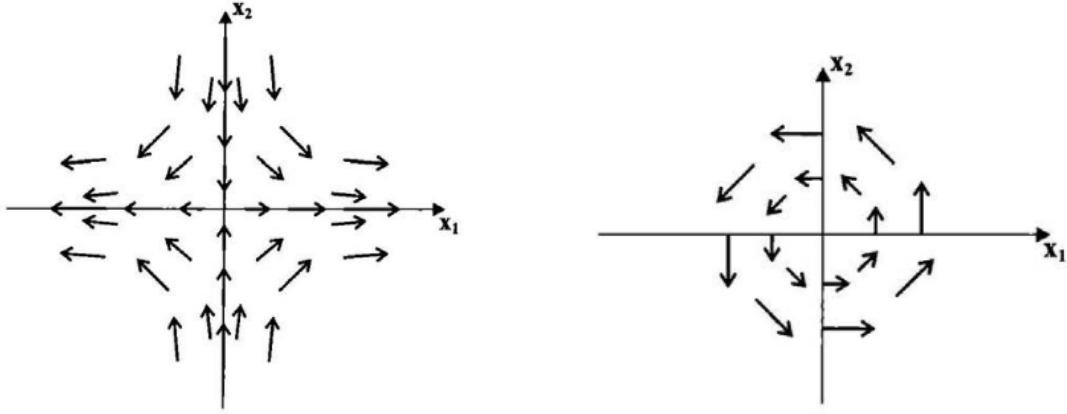
297. ábra. A C_{ik}^{(1)} és C_{ik}^{(2)} tenzorok által leírt sebességmezők. Az első egy táguló/összehúzódó mezőt ír le, míg a második egy forgó mezőt.
