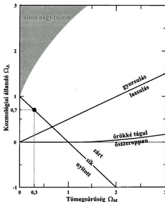
299. ábra. Az univerzum tágulásának időfejlődése különböző kozmológiai paraméterek mellett.
