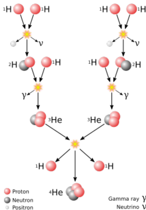
311. ábra. A proton-proton láncreakció folyamata.
