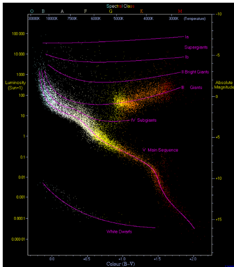
309. ábra. Egy tipikus Hertzsprung-Russell diagram a Hipparcos és a Gliese katalógusokból összeszedett minted 22000 csillagról. Az MK spektrum és luminozitás osztályok is fel vannak tüntetve, mindkettő napegységekben.
