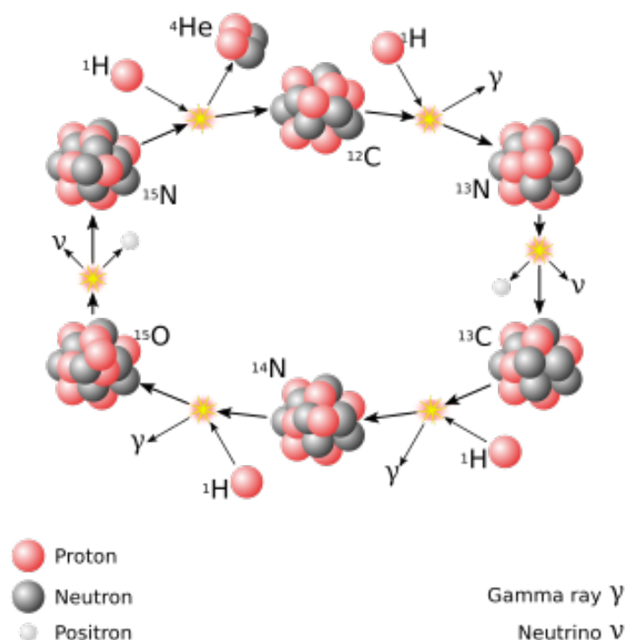
312. ábra. A CNO ciklus folyamata.
