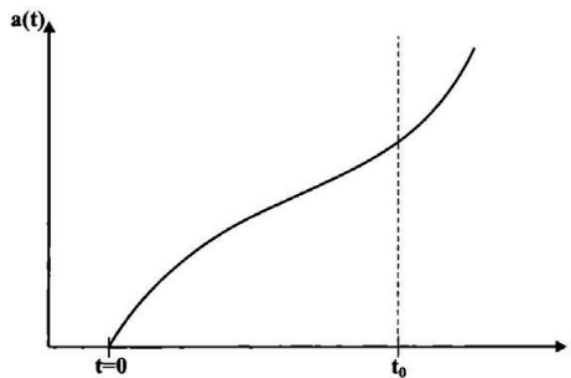
302. ábra. Az univerzum tágulási paraméterének időfejlődése jelenlegi tudásunk szerint. Ez az ábra jól mutatja, hogy az univerzum tágulása a múltban lassult, majd a kozmológiai állandó dominanciája miatt a közelmúltban gyorsuló fázisba lépett.
