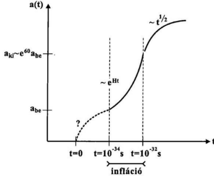
305. ábra. A skálafaktor időbeli változása az inflációs modellben.
