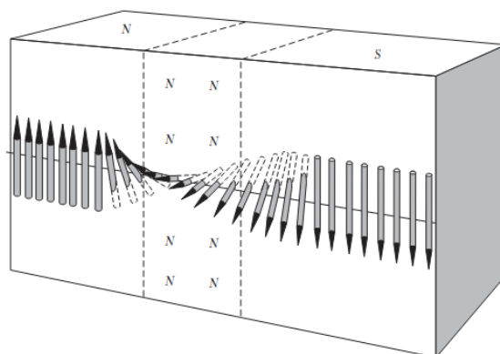
262. ábra. Mágneses domain fal illusztrációja.
